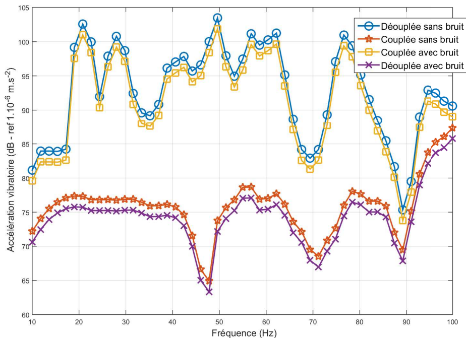
FIGURE 4.4 – Bruitage de l'accélération vibratoire du point de mesure 1 d'une plaque couplée et découplée du sol
