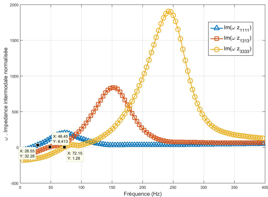
FIGURE 2.10 – \omega \cdot Partie imaginaire de l'impédance intermodale de rayonnement vibratoire normalisée dans la cas d'une structure de 6m de large et 6m de long.
