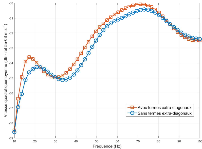
FIGURE 2.5 – Influence des termes extra-diagonaux sur la vitesse quadratique moyenne dans le cas d'un couplage plaque/sol monocouche ( c_p = 600m.s^{-1} , \eta_p = 0.02, c_s = 160m.s^{-1} , \eta_s = 0.02 et \rho = 1200Kg.m^{-3} )
