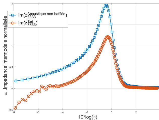
FIGURE 2.26 – Comparaison de la partie imaginaire des impédances intermodales de rayonnement des modes (3,3) dans le cas d'un couplage élastique et dans le cas d'un couplage acoustique non baffé
