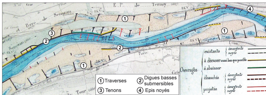
Figure 2.2. Etat de l'endiguement du Rhône en 1891 entre Grigny et Ternay (tronçon de Pierre-Bénite). Cette planche illustre parfaitement la complexité des travaux de correction du fleuve entrepris en aval de Lyon et l'approche empirique de gestion et de calibration des infrastructures qui existait alors (tiré des plans de "Travaux de parachèvement et de premier entretien entre Lyon et Saint Vallier, Kilomètre 0 et 75.650, service spécial du Rhône, 1891).
