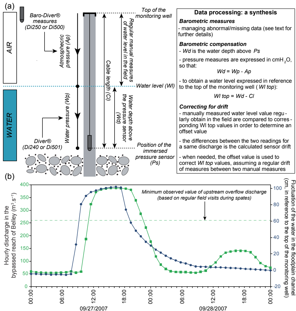
Figure 2.10. Suivi automatisé et continu des hauteurs d'eau dans les bras morts à partir des sondes Diversers®. (a) Principes de mesures et synthèse de la chaîne de traitements réalisés pour obtenir les niveaux d'eau dans les bras. (b) Illustration des données obtenues à un pas de temps horaire. Ici, un hydrogramme de crue sur le bras restauré des Luisettes. Les débits horaires sont fournis par la CNR.
