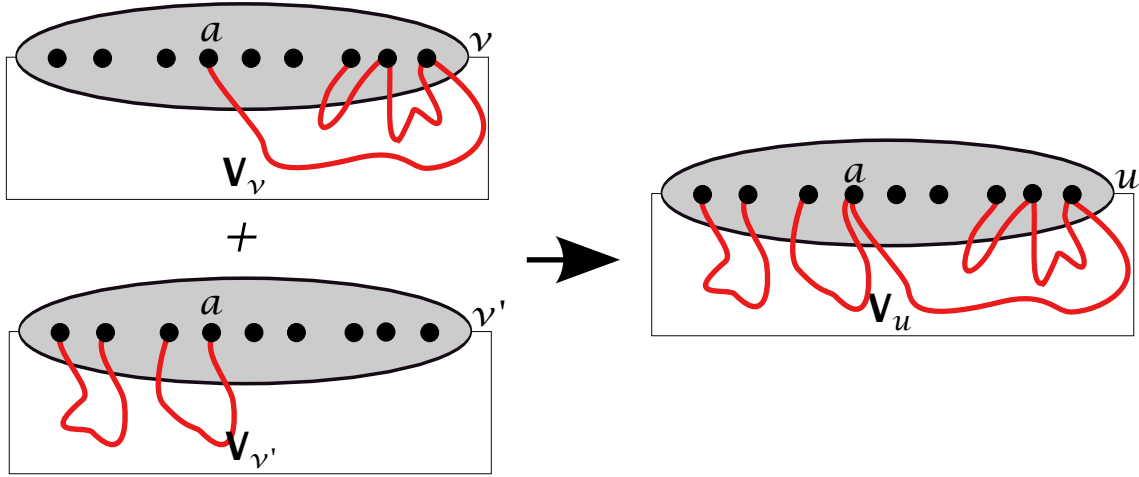
FIGURE 3.9 – u est un nœud joint - L'union des deux solutions aux nœuds v et v' est une solution au nœud u si la transition de centre a est autorisée.
