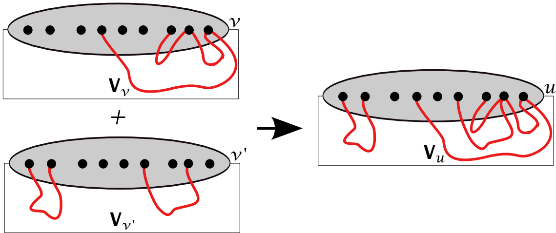
FIGURE 3.10 – u est un nœud joint - L'union des deux solutions aux nœuds v et v' n'est pas une solution au nœud u car elle a un sommet de degré 3.
