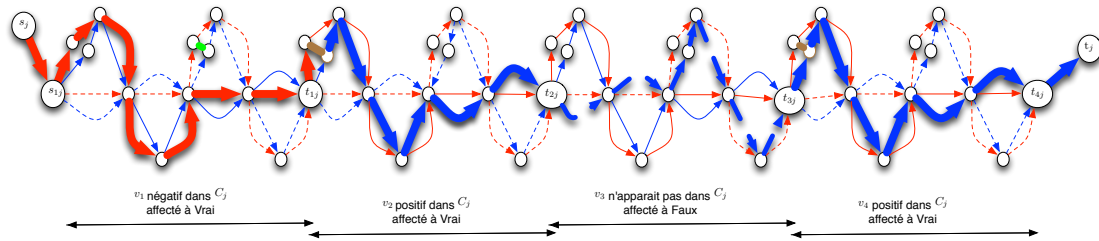
FIGURE 4.2 – Cas j impair. Le clause-graphe G_j pour une clause C_j = \bar{v}_1 \vee v_2 \vee v_4 d’une formule à 4 variables. Le chemin en gras correspond à une affectation à Vrai de v_1, v_2 et v_4 , et à Faux de v_3 .
