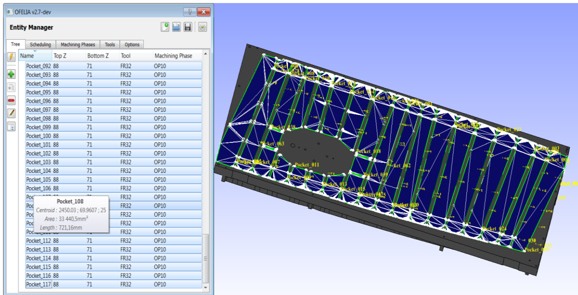
Figure 3.38 : Entités détectées
