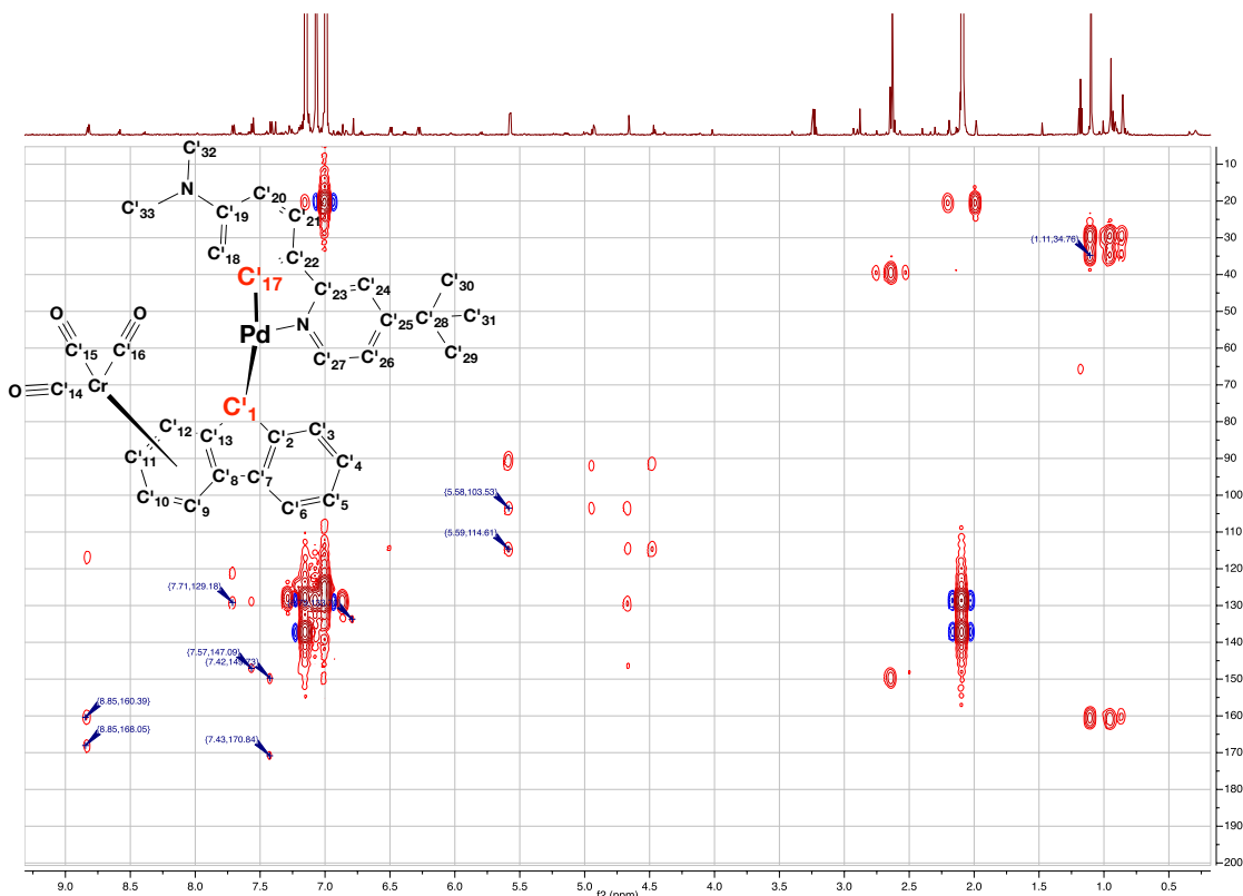
Tol – HMBC – (600 Mhz, 151 Mhz) – 223 K.
