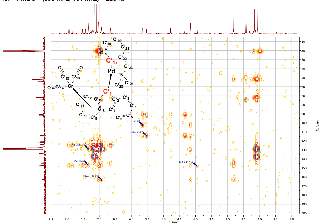
Tol - HMBC - (600 Mhz, 151 Mhz) - 223 K.
