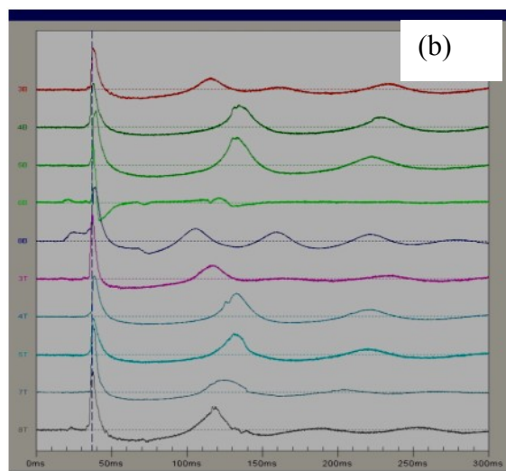
Figure II.5 : Caractéristiques techniques du dispositif source « Pic ». Configuration des canons à air ; seuls les 10 canons en verts sont actifs, les autres peuvent servir comme lest, mais également peuvent remplacer les canons défectueux ; (b) fenêtre de contrôle des 10 signaux source synchronisés sur le premier pic (trait en pointillés).
