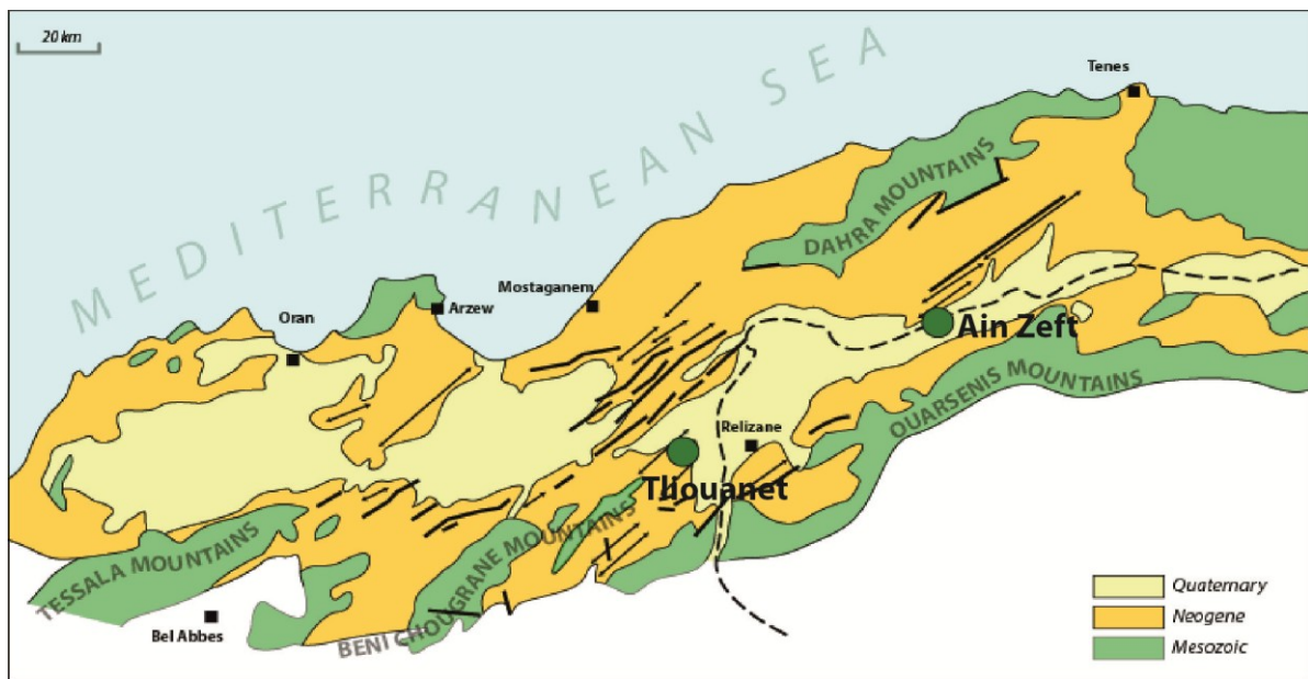
Figure. V.15 : Carte géologique simplifiée du bassin du Chelif, montrant la position des gisements de Aïn Zeft et Tliouanet. (Document Sonatrach).
