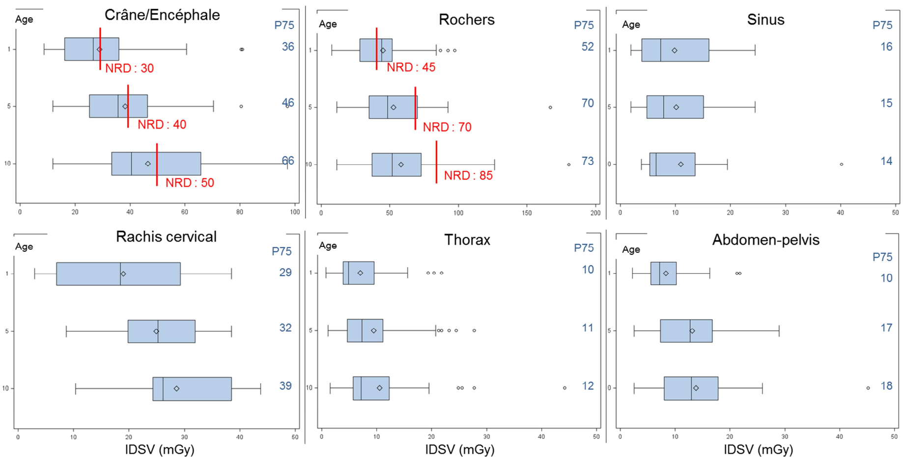
Figure 13 Indices de dose en scanographie dans le volume (IDSV) associés à des protocoles utilisés dans 22 services de radiologie entre 2000 et 2011 et niveaux de référence diagnostique (NRD) en France en pédiatrie 26
