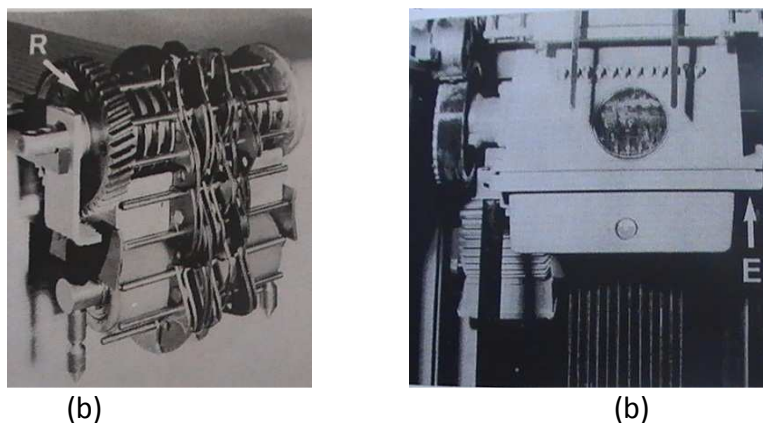
Figure A2. 4: Montage chaîne-dessin
