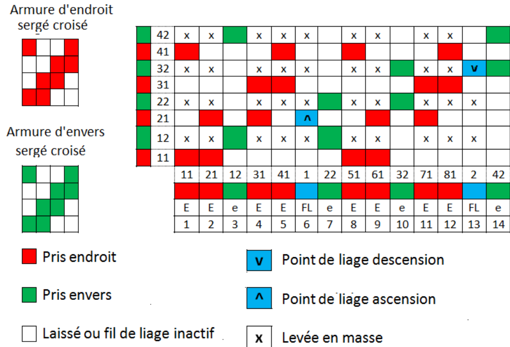
Figure 2. 5: Double étoffe liée par une chaîne de liage
