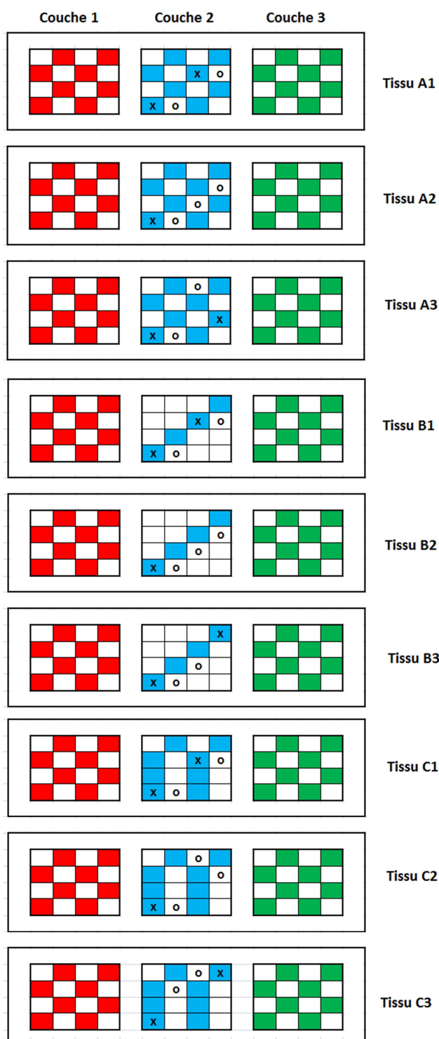
Figure 5. 24: Les armures définitives
