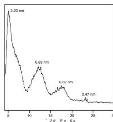
Fig. 5.2 – Exemple de diagramme de diffraction obtenue pour une poudre de fagots de nanotubes d'imogolite AlSi. D'après Tanni et coll. [101].
