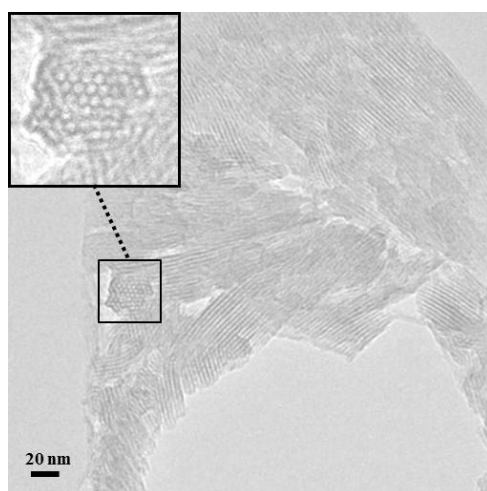
Fig. 5.11 – Image TEM d'une poudre déshydratée de nanotubes d'imogolite AlGe mono-pareil ( C_{Al} = 1 \text{ mol.L}^{-1} et R(OH/Al) = 2 ) emprisonnée entre deux résines (voir détails de préparation dans chapitre 2). Le zoom montre une coupe orthogonale à l'axe d'un fagot de nanotubes.
