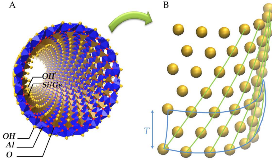
Fig. 4.2 – (A) Image d'un nanotube d'imogolite AlSi(Ge) mono-paroi, contenant L entités Si_xGe_{1-x}O_3Al_2(OH)_4 sur sa circonférence. (B) Couche formée par les atomes de silicium (germanium). L'encart bleu indique la maille, avec la période de répétition T suivant l'axe du nanotube, et les lignes vertes indiquent l'arrangement des atomes de silicium (germanium) sous forme d'hélices sur la surface de la couche atomique. Il y a L hélices parallèles sur cette surface.
