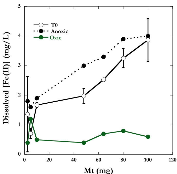
Figure IV.17 : Evolution de la concentration en Fe(II) dissous à T 0 et avant l'étape de désorption sous conditions anoxiques et oxic (2x15 min de bullage d'air) en fonction de la quantité de nano-magnétite.
