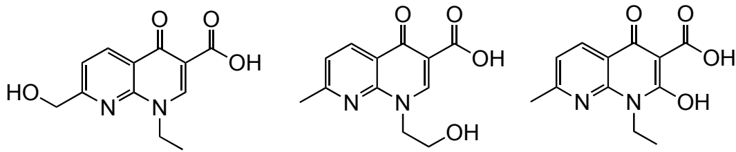
Figure I.6 : Différents isomères de position issus de l’hydroxylation de NAL.
