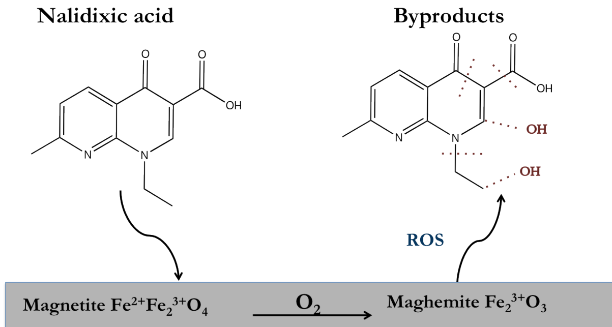
Figure IV.26 : Schématisation de la dégradation de l'acide nalidixique par la magnétite en présence d'oxygène dissous.
