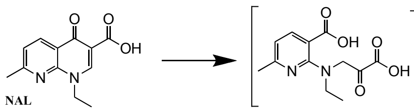
Figure I.8: Initiation de l'ouverture du cycle proposé par Fan et al. (2013).
