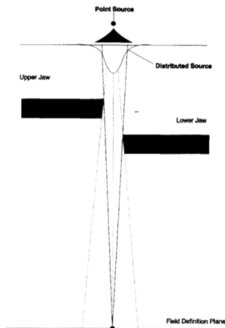
FIGURE 1.5 – Modèle multisource décrit dans [Dunscombe and Nieminen, 1992]. Point source : une source ponctuelle de photons directs. Distributed source : un plan source de photons diffusés par les premières composantes de la tête d'irradiation rencontrées (collimateur primaire et filtre égalisateur en triangle en noir) muni d'une distribution d'intensité Gaussienne. Jaws : les mâchoires ou collimations secondaires définissent la portion visible du plan des photons diffusés.
