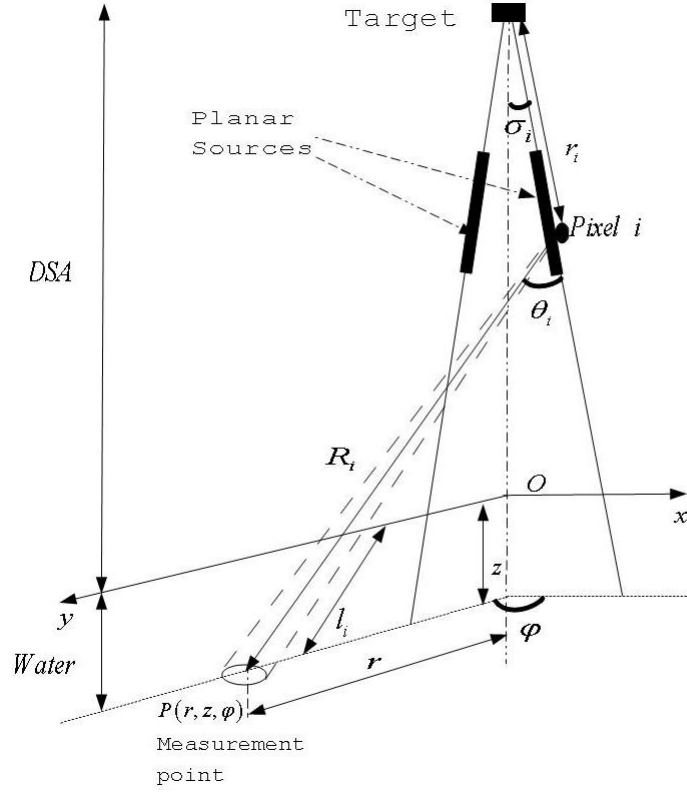
FIGURE 1.8 – Termes géométriques utilisés dans l’expression du modèle final de l’équation 1.9
