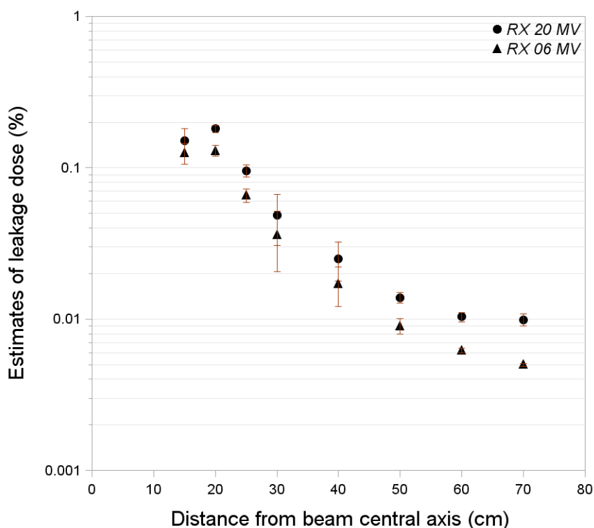
FIGURE 1.9 – Estimation des doses du rayonnement de fuite (paramètre \lambda(r, \varphi, z) de l'équation (1.3)) pour l'accélérateur linéaire Varian Clinac 2300 C/D opérant à 6 et 20 MV RX, respectivement. Les doses sont données en pourcentage de la dose à la profondeur de la dose maximale à l'axe du faisceau.
