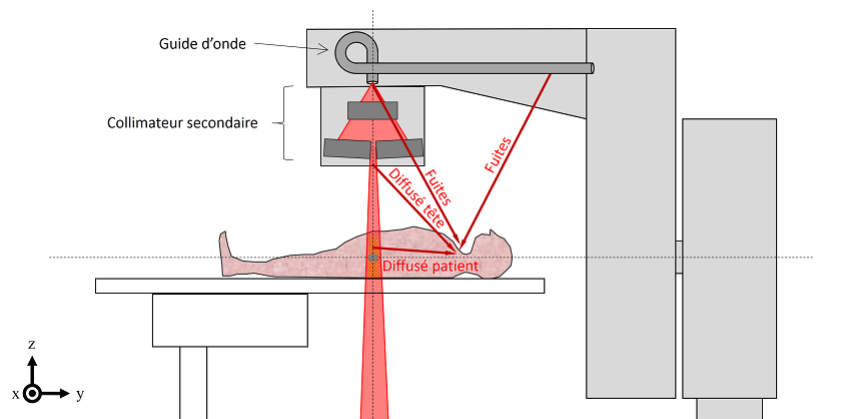
FIGURE 1.4 – Les composantes de la dose hors champ. Un repère en bas à gauche indique la convention adoptée en radiothérapie pour définir l'espace. L'origine de ce repère est l'isocentre de l'appareil, défini ici par l'intersection de l'axe central du faisceau et celui de rotation du statif de l'appareil, tous deux représentés sur la figure par des lignes en pointillés.
