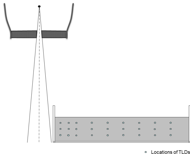
FIGURE 1.6 – Dispositif expérimental utilisé pour la mesure de la dose due aux rayonnements de diffusions collimateurs et fuites.
