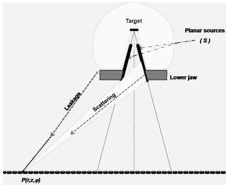
FIGURE 1.7 – Une représentation schématique de la source surfacique \mathcal{S} , du blindage linéaire de la tête de l'accélérateur ainsi que des mâchoires inférieures du collimateur secondaire.
