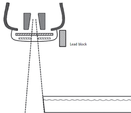
FIGURE 1.2 – Dispositif expérimental utilisé dans [Ruben et al., 2014] permettant de ne mesurer que la composante diffusé tête (ou collimateur) de l’accélérateur
