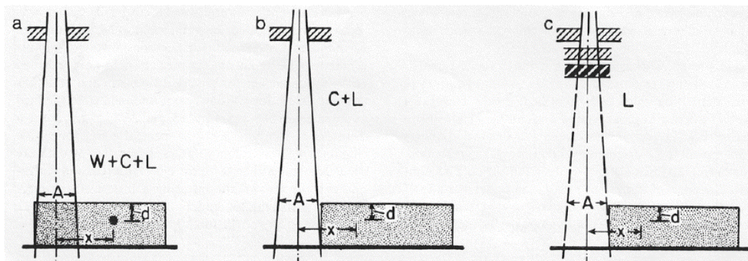
FIGURE 1.1 – Mises en place expérimentales utilisées dans l'article de Kase et al. [Kase et al. , 1983]. W , est le diffusé patient, C , le diffusé tête, et L , les fuites. Pour un champ carré de côté A , le point de mesure est à une distance x de l'axe du faisceau, et à une profondeur d .
