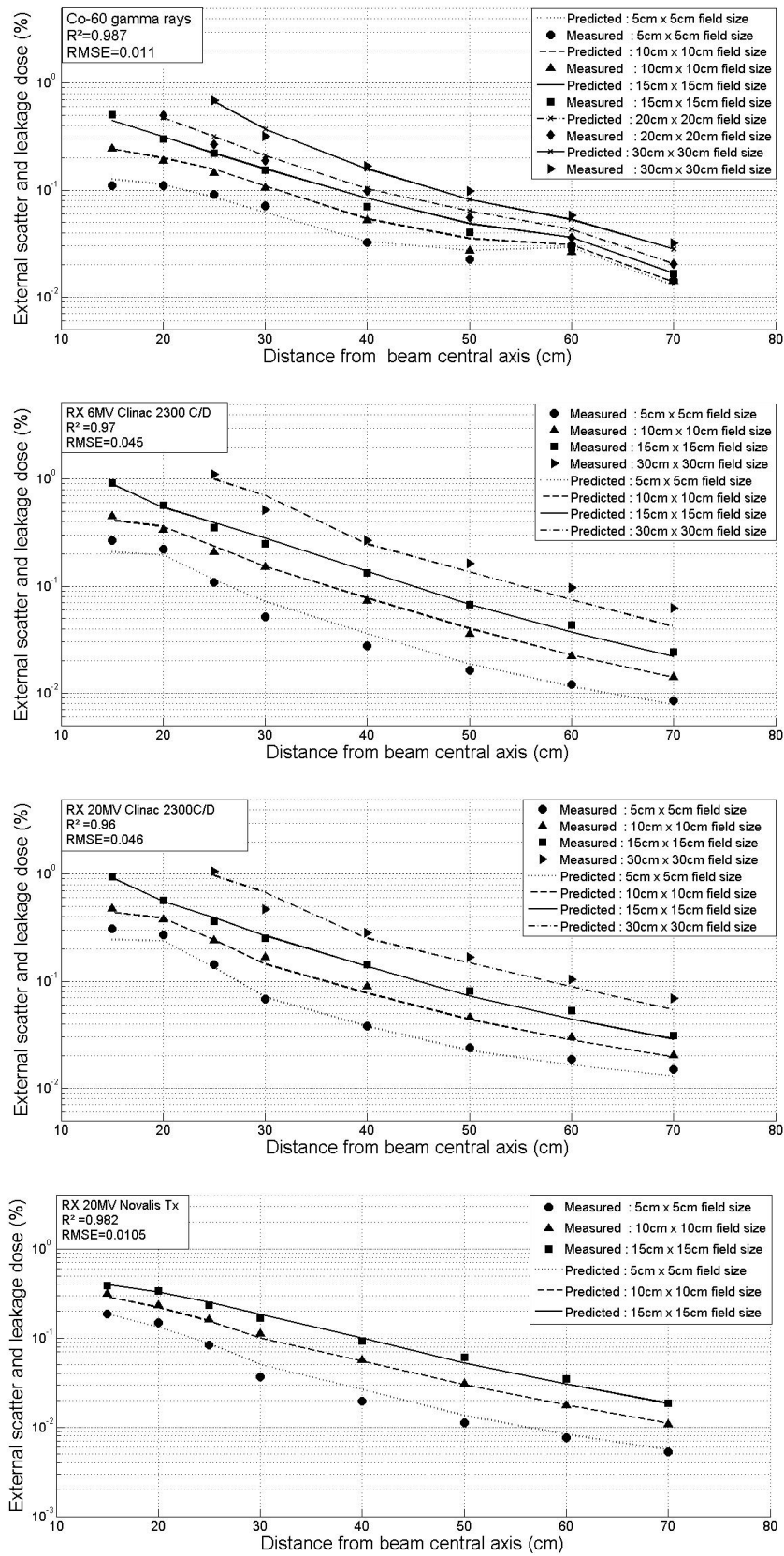
FIGURE 1.10 – Comparaison des profils de doses à distance mesurés et calculés, à 10cm de profondeur, pour différents appareils et différentes conditions d’irradiation.
