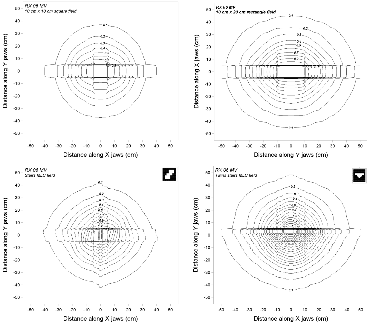
FIGURE 1.11 – Isodoses calculées pour différentes tailles et formes de champs représentés en haut à gauche. Les doses sont données en pourcentage de la dose maximale à l'axe du faisceau. Les calculs sont effectués pour Varian accélérateur linéaire Clinac 2300 C/D opérant à 6 MV.
