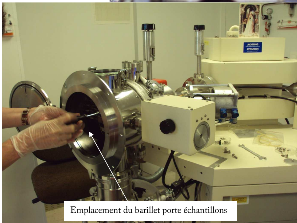
Barillet à Double filament Re
