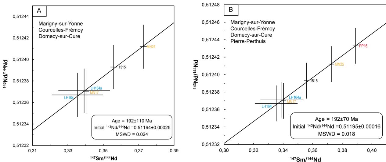
Figure 6 : (A) Diagramme errorchrone des échantillons de fluorine géodique de Marigny-sur-Yonne, Courcelles-Frémoy et Domecy-sur-Cure ; (B) Diagramme errorchrone des échantillons géodique incluant l'échantillon de Pierre-Perthuis PP16
