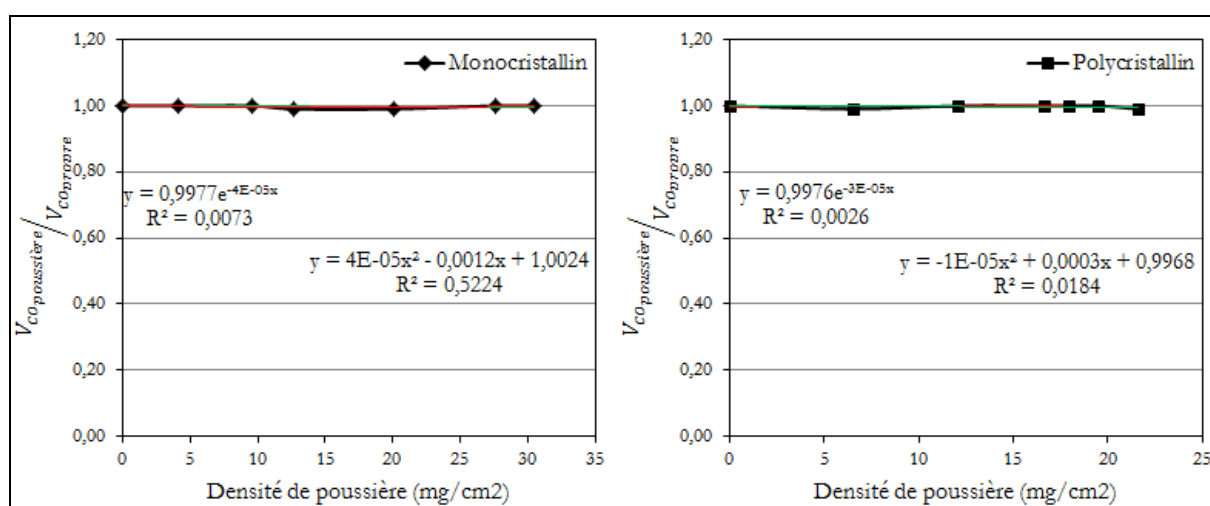
Figure IV- 15. Corrélation de la tension en circuit ouvert normalisée avec la densité de poussière par les régressions exponentielle et polynomiale.
