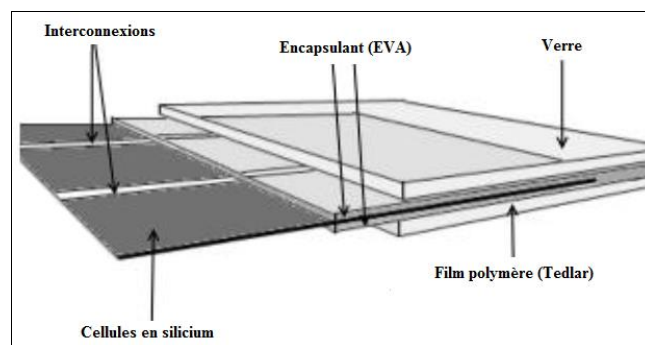
Figure II- 1. Les différents composants du module photovoltaïque soumis à la dégradation.
