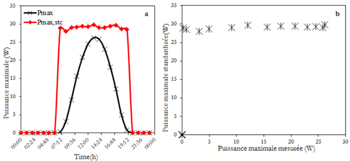
Figure III- 18. Comparaison (a) et corrélation (b) entre la puissance maximale mesurée et standardisée.
