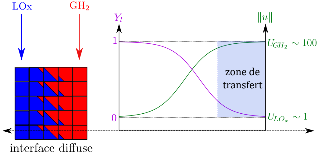
FIGURE 10.5 – Représentation schématique des profils de vitesse et de fraction massique de liquide à travers l'interface diffuse.
