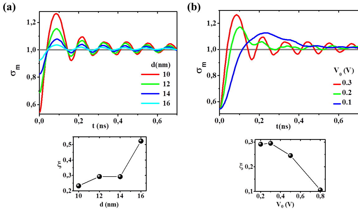
Figure V.12 : Evolution temporelle de l'écart type normalisé de la distribution de l'aimantation longitudinale \sigma_m durant le dépiégage de la paroi transverse (a) de constriction de diamètres d différents soumise à la tension V_0=0,3\text{V} ( U_T=203\text{m/s} , j^e=4\cdot 10^{12}\text{A/m}^2 , I=1,26\text{mA} ), (b) d'une constriction de diamètre d=10\text{nm} soumise à différentes tensions. Les encarts représentent l'évolution de l'estimation du facteur d'atténuation \xi en fonction de d et V_0 .
