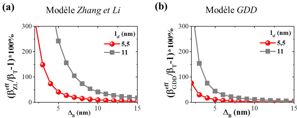
Figure II.11 : Ecart relatif entre le paramètre de non-adiabaticité effectif et la valeur théorique pour une distribution de Bloch 1D en fonction de la largeur de paroi et pour l_{sf}=5,5\text{nm} et l_{sf}=11\text{nm} (a) dans le modèle de Zhang et Li \beta_{ZL}^{eff1D} pour avec l_{sd}=1,1\text{nm} (b) dans le modèle GDD \beta_{GDD}^{eff1D} pour l_p=1\text{nm} . L'effet de la diffusion est d'autant plus marquée que la largeur de paroi est petite et l_{sf} est grand. (a) et (b) sont tracés pour P=0,76 , C_0=3,436 \cdot 10^6 [ \Omega\text{m} ], D_0=2,3 \cdot 10^{-3}\text{m}^2/\text{s} , V_0=0,1V .
