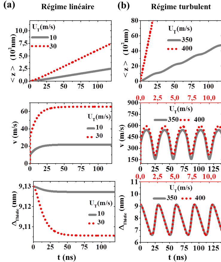
Figure IV.11 : Mise en évidence des régimes (a) laminaire et (b) précessionnel suivant la position moyenne de la paroi sur l'axe z (1 ère ligne), la vitesse moyenne de propagation (2 ème ligne) et la largeur de paroi \Delta_{\text{Thiele}} (3 ème ligne) en fonction du temps. Les graphes sont tracés pour une paroi transverse dans un ruban de permalloy de largeur w=120\text{nm} et d'épaisseur d=5\text{nm} dans le modèle non local de Zhang et Li pour l_{sf}=5\text{nm} .
