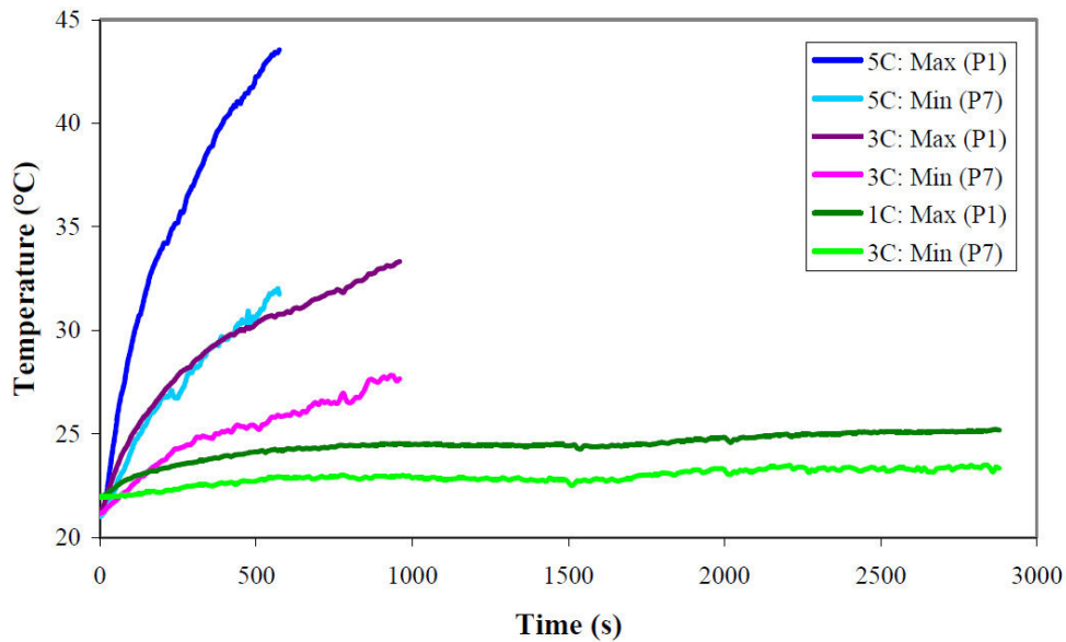
Figure 3. Comparaison de max et min température pour différents taux de décharge avec une vitesse d'air de refroidissement de 2 m/s.
