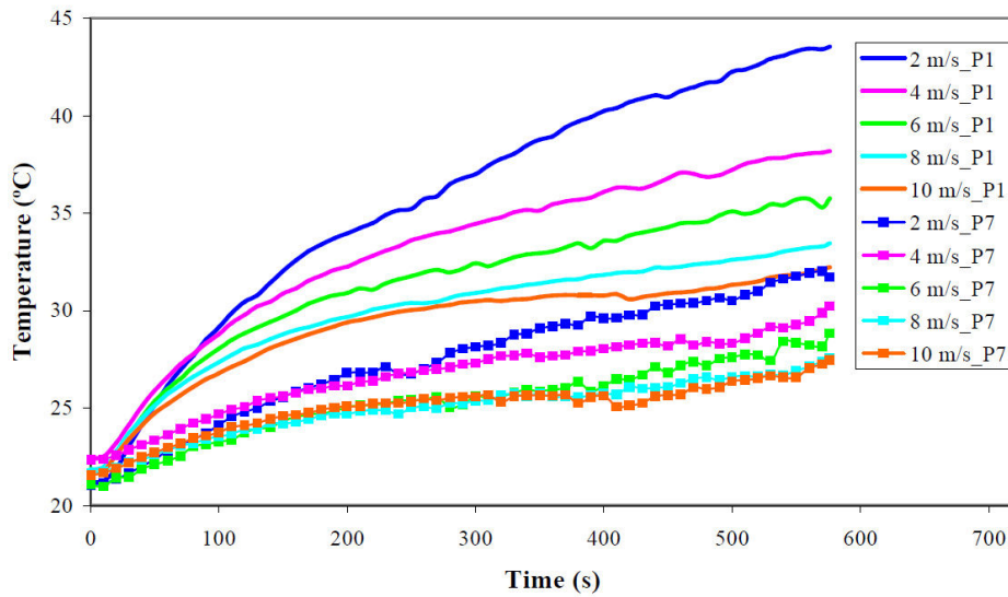
Figure 4. La température de la surface 1R (P1 et P7) à cinq vitesses d'air de refroidissement différent au taux de décharge de 5C.
