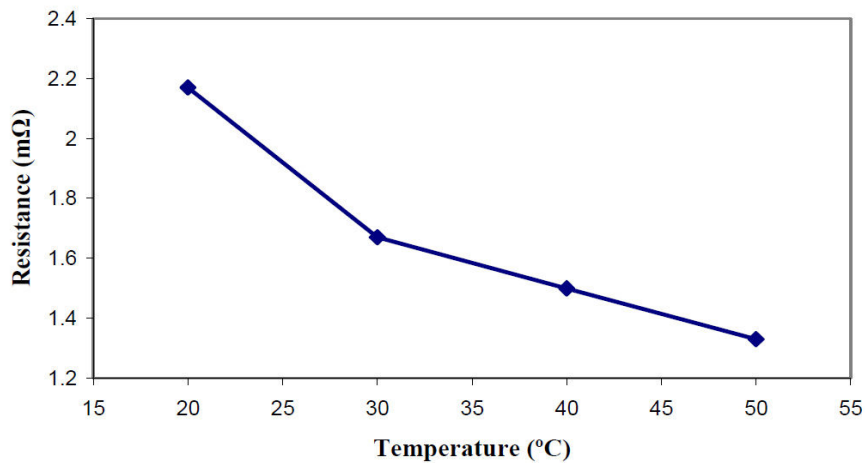
Figure 6. La résistance interne de la batterie en fonction de la température.
