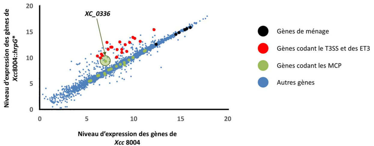
Figure 3.1 : Niveaux de transcription des gènes de Xcc 8004 . Les niveaux de transcription de tous les gènes du génome de Xcc 8004 et de Xcc8004::hrpG* (bleu), des gènes de ménages (noir), des gènes codant des effecteurs de type III (ET3) et la structure du système de sécrétion de type III (T3SS) (rouge), et ceux codant les MCP (vert) ont été déterminés grâce à une analyse RNAseq de Xcc 8004 et de Xcc8004::hrpG* .
