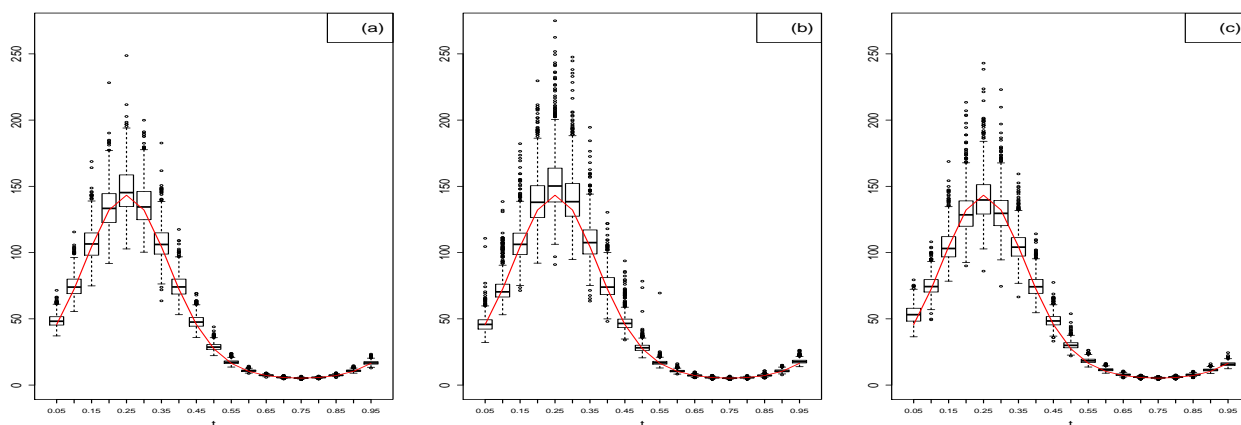
Figure III.9 – Boîte à moustaches des estimateurs de F_t^{-1}(0.999) pour N_{MC} = 1000 en choisissant la taille de la fenêtre h par (a) le choix h = h_{opt} ; (b) la méthode adaptative et (c) la méthode de la validation croisée.
