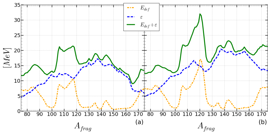
FIGURE 3.27 – Énergie de déformation (courbe orange), d'excitation intrinsèque (courbe bleue) et d'excitation totale (courbe verte) en fonction de la masse du fragment pour la réaction ^{235}\text{U}(n_{thr}, f) (a) et ^{252}\text{Cf}(sf) (b) dans le cas d'une distribution de charge issue des calculs HFB.
