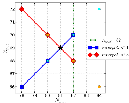
FIGURE C.3 – Représentation des différentes possibilités pour le calcul de la masse interpolée quadratiquement du ^{150}\text{Tm}_{81} en présence d'un nombre magique ( N_{nucl} = 82 ).
