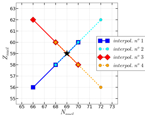
FIGURE C.2 – Représentation des différentes possibilités pour le calcul de la masse interpolée quadratiquement du ^{128}\text{Pr}_{69} (étoile noire).
