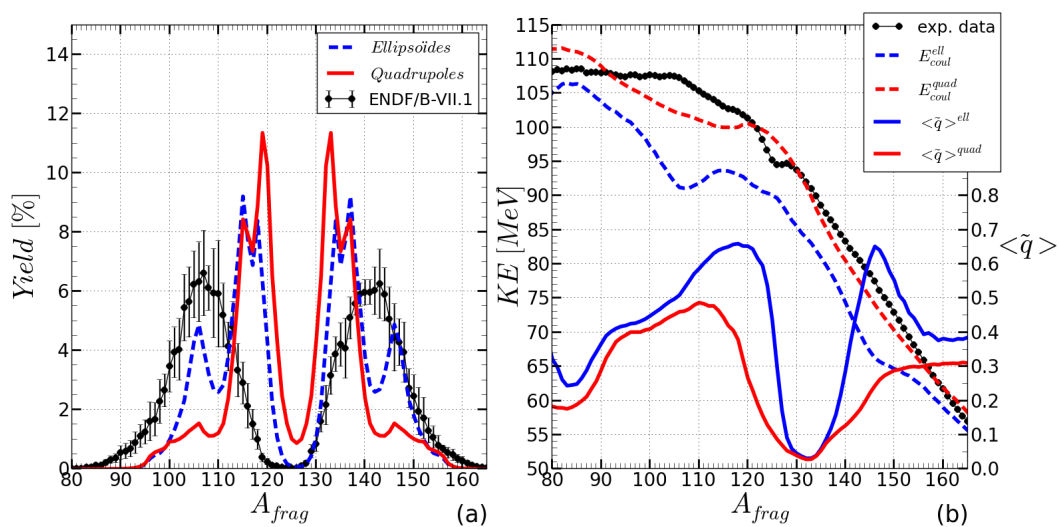
FIGURE 3.8 – Rendements isobariques (à gauche) ou distribution en énergie cinétique et déformation moyenne (à droite) pour la réaction ^{252}\text{Cf}(s, f) pour les deux formes de surface, comparés avec les données évaluées [24] ou expérimentales [27].
