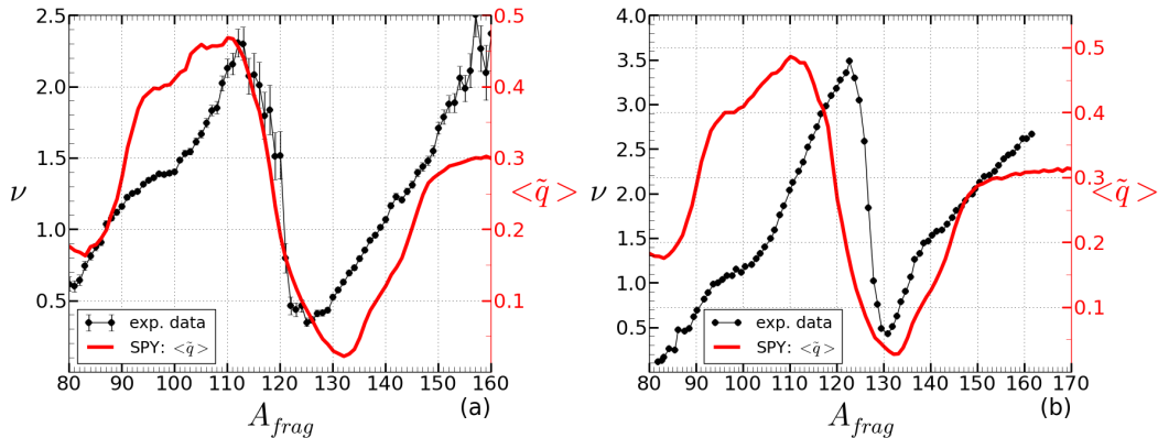
FIGURE 2.7 – Comparaison entre la distribution de neutrons évaporés et la déformation de la moyenne ( \bar{q} ) ( A_{\text{frag}} ) en fonction de la masse A_{\text{frag}} du fragment pour la réaction ^{235}\text{U}(n_{\text{th}}, f) (a) et pour la réaction ^{252}\text{Cf}(sf) (b). Les distributions de neutrons évaporés expérimentaux est issues de [28] (a) et [27] (b)
