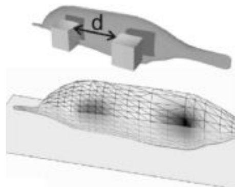
(b) Calcul numérique de l'image électrique de deux cubes sur un avatar numérique d'un PFE. Image tirée de [42].
