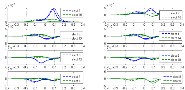
(b) Mesures effectuées, en ampères, sur les électrodes de la sonde. Les traits continus représentent les résultats BEM, tandis que les traits discontinus ceux du simulateur.
