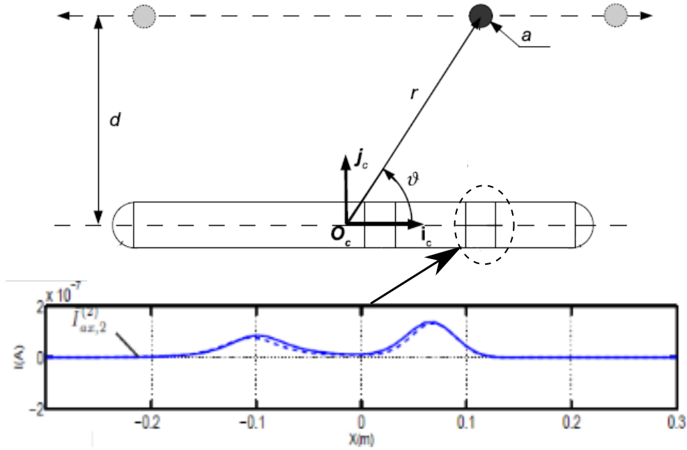
FIGURE 1.9 – Une sphère se déplace parallèlement à l’axe de la sonde élancée. Le courant est mesuré sur la bague \mathcal{E}_2 tout au long du déplacement de la sphère, créant ainsi une image électrique de cette dernière.
