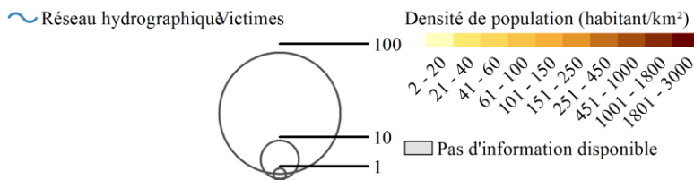
Figure V.20 Densité de population (recensement de 1926) et nombre de décès des inondations de mars 1930 (Source : Recensements issus de site du site des « Villages de Cassini aux communes d'aujourd'hui 52 )
