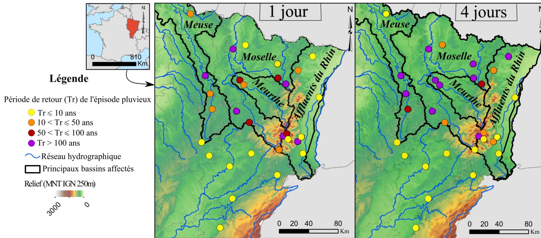
Figure IV.12 Périodes de retour des précipitations du 26 au 30 décembre 1947 (cumuls sur 1 jour et 4 jours)
