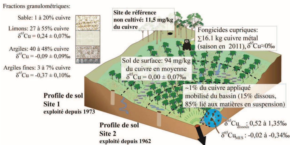
Figure 2 : La répartition du cuivre dans les fractions granulométriques du sol en surface au points d'échantillonnage ('Site 1' et 'Site 2') et leur rapport isotopique, le bilan du cuivre au niveau du bassin versant du Hohrain (Rouffach, France) : le cuivre cumulé appliqué pendant la saison d'application en 2011 ainsi que le rapport isotopique moyen du cuivre dans les fongicides cupriques, la concentration en cuivre et son rapport isotopique dans sols en surface du bassin versant et la répartition du cuivre dans la lame ruisselante à l'exutoire du bassin versant ainsi que les rapports isotopique.
