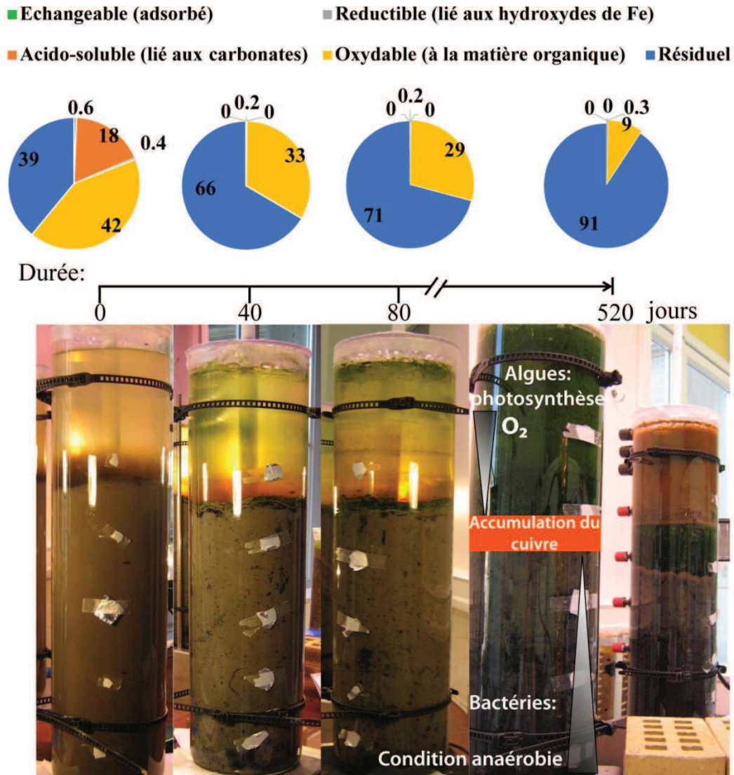
Figure 4 : L'évolution visuelle des colonnes de Winogradsky et le « vieillissement » du cuivre dans les sédiments mis en évidence par le changement de la répartition du cuivre entre les différentes phases dans les sédiments (i.e., carbonates, hydroxydes de fer, matière organique, minéraux silicatés)
