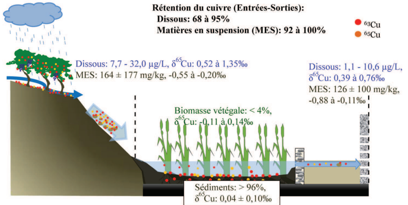
Figure 3 : Les concentrations et les rapports isotopiques du cuivre en entrée et en sortie du bassin de rétention, ainsi que la répartition du cuivre à l'intérieur du bassin à Rouffach
