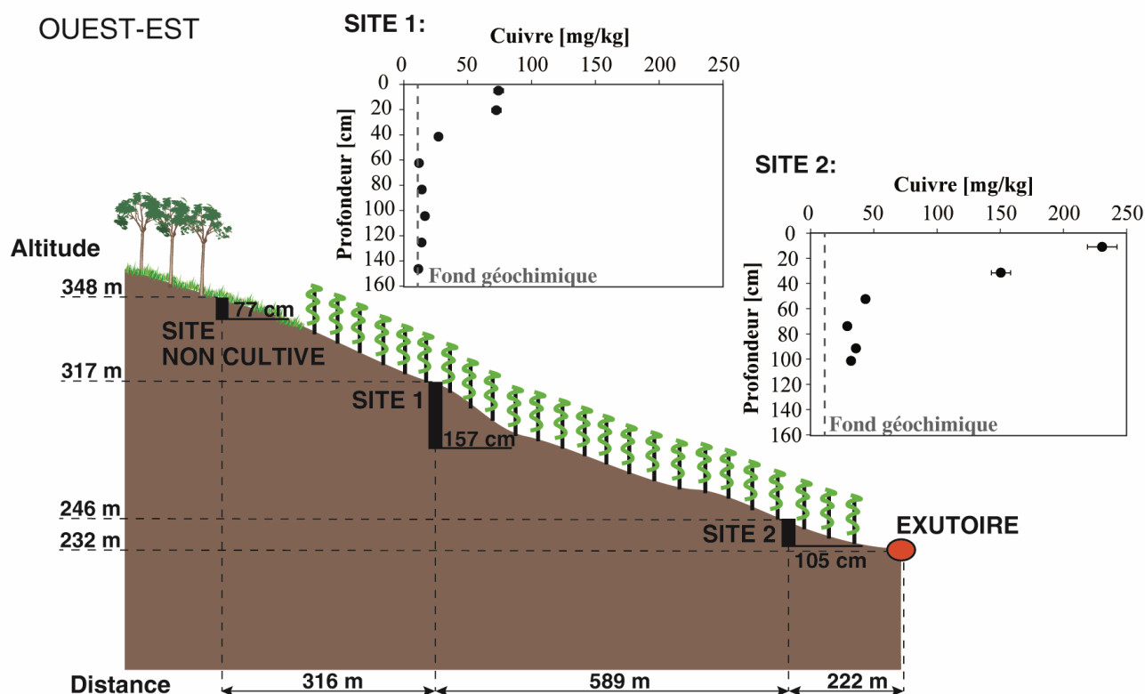
Figure 3 : Les concentrations en cuivre des sols viticoles en fonction de la profondeur aux sites d'échantillonnage ('Site 1' et 'Site 2') dans le bassin versant du Hohrain (coupe ouest-est), et la concentration en cuivre du sol local non cultivé ('fond géochimique du cuivre').
