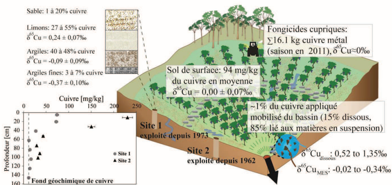
Figure 2 : Signatures isotopiques des sources, la répartition du cuivre dans les fractions granulométriques du sol, la signature moyenne des sols de surface et la répartition du cuivre dans la lame ruisselante à l'exutoire du bassin versant viticole à Rouffach
