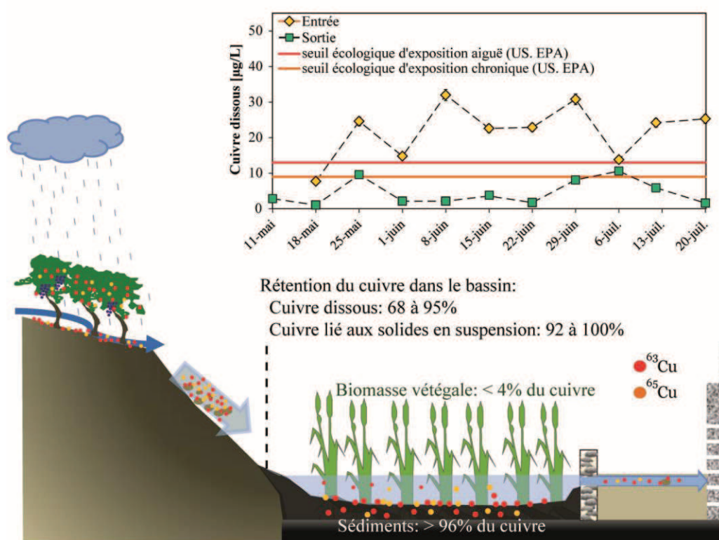
Figure 4 : Répartition du cuivre, ainsi que sa répartition à l'intérieur du bassin d'orage à Rouffach (US. EPA : Agence Américaine de la Protection de l'Environnement).
