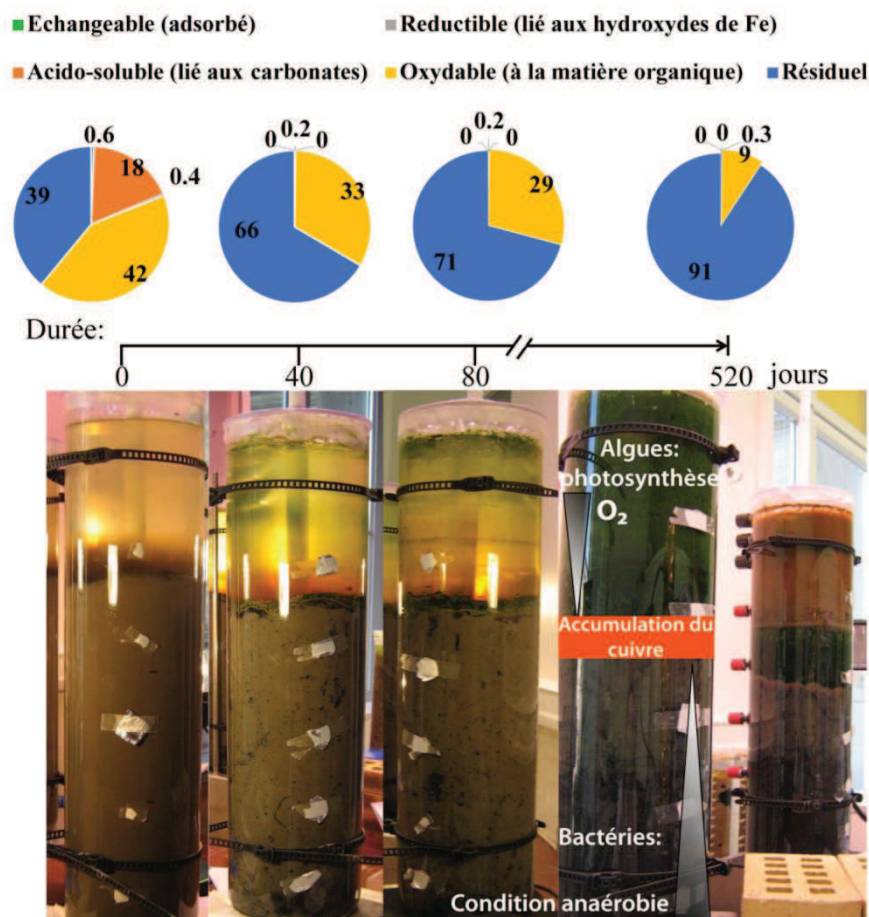
Figure 5: Evolution des colonnes de Winogradsky et évolution du cuivre dans les sédiments mis en évidence par le changement de la répartition du cuivre (%) entre les différentes phases dans les sédiments (i.e., carbonates, hydroxydes de fer, matière organique, minéraux silicatés)
