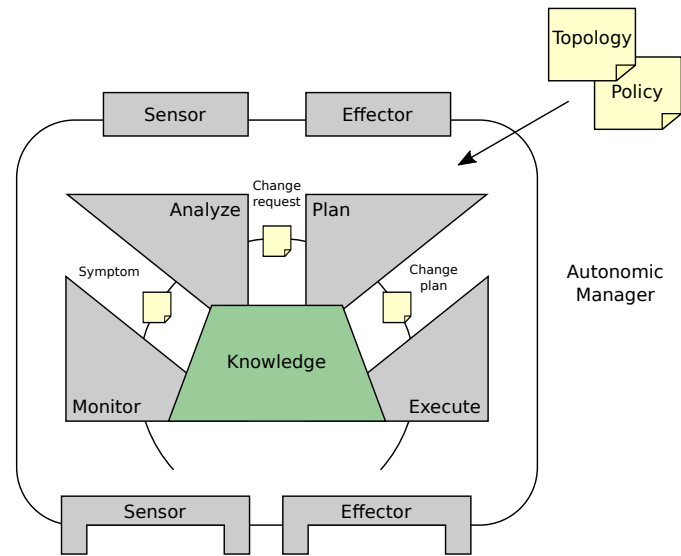
FIGURE 6.2 – Représentation d’une boucle autonome Définie par [KC03].
