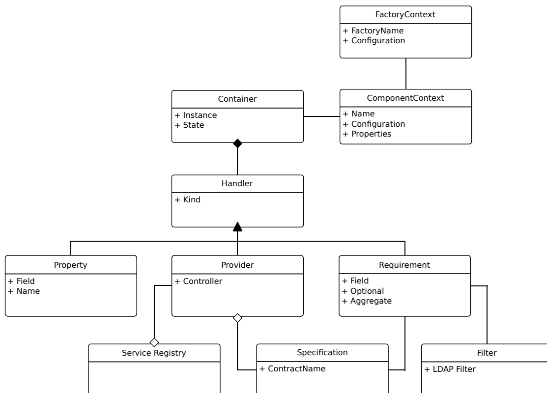
FIGURE 3.2 – Métamodèle iPOPO
