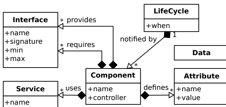
FIGURE 2.6 – Modèle de composant Fraclet
