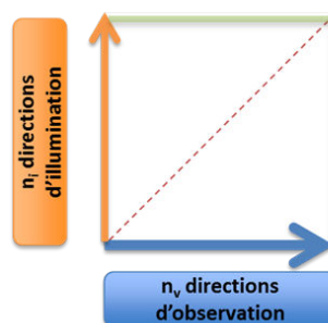
FIGURE 2.9 – Configurations mesurées par le dispositif Mesura, ici identifiées par la droite rouge, la droite verte correspond à leur principe inverse.
