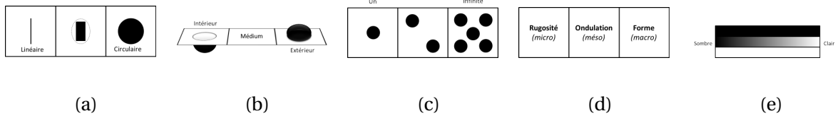
FIGURE 3.4 – Les cinq lois d'apparence pour décrire les anomalies de la norme ISO-8785 (1998).
