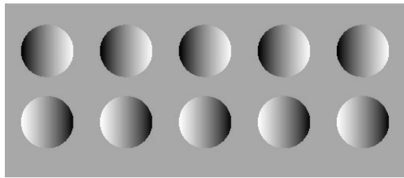
FIGURE 3.22 – Illusion d'optique des bosses et des creux.
