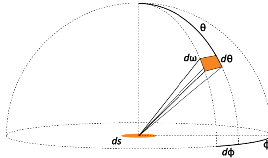
FIGURE 2.17 – Illustration de la projection d'un angle solide de surface élémentaire dS sur la sphère de rayon x .
