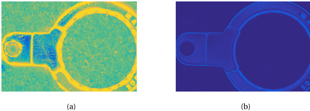
FIGURE 4.17 – Images résultat, respectivement du maximum et du minimum, des informations des P photographies
