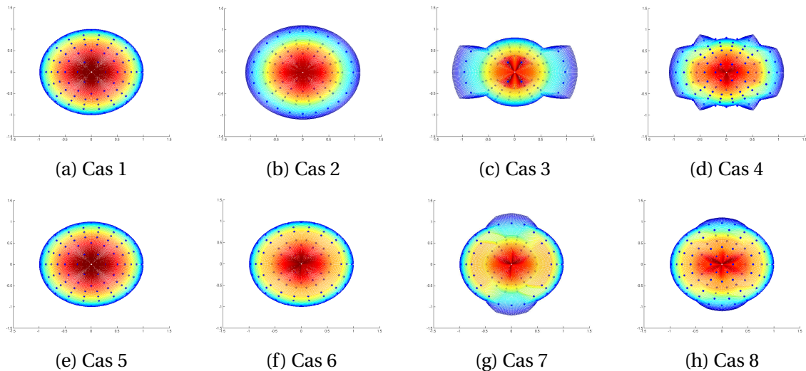
FIGURE 4.21 – Représentation des BHF de l'homogénéité dans le plan de référence X-Y, suivant les cas illustrés par la figures 3.12 et 3.13
