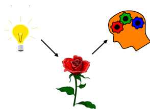
FIGURE 2.2 – Le schéma d'un problème de vision selon la Commission Internationale de l'Eclairage (CIE).
