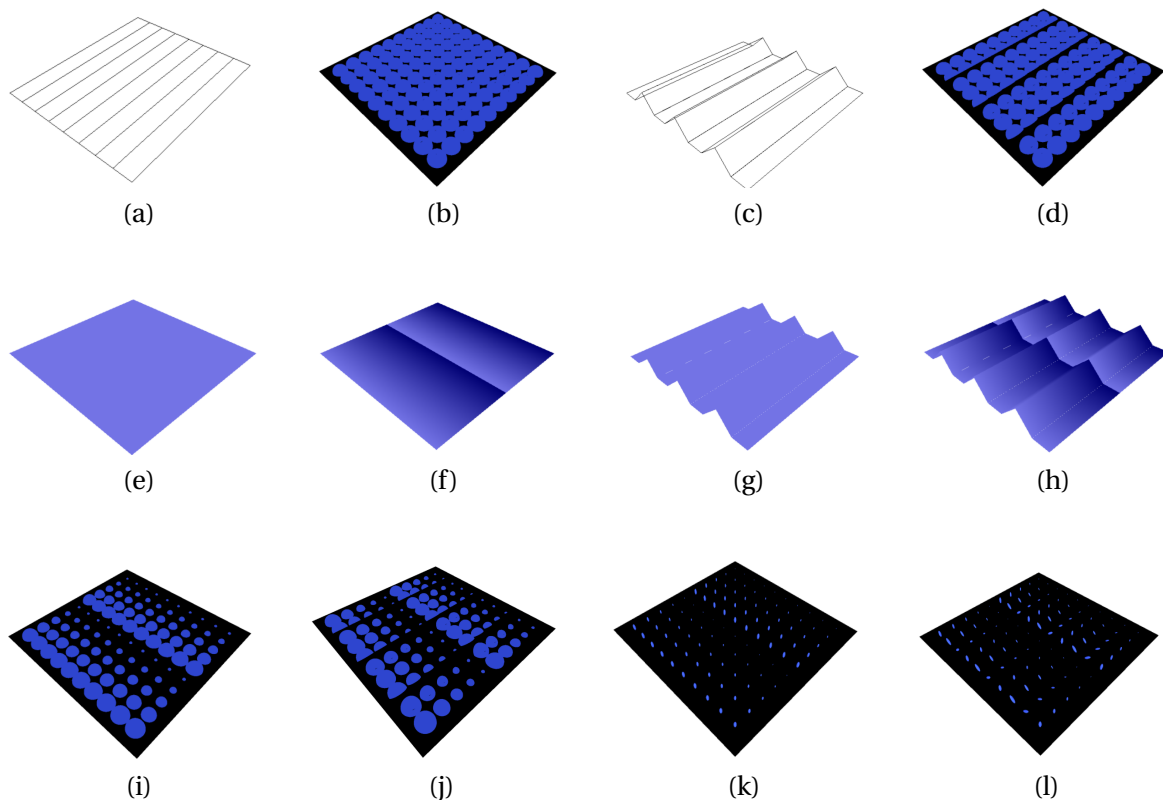
FIGURE 3.13 – Représentation de l'apparence d'une surface et de champs de BRDF associés, pour un champ d'observation de 10 pixels par 10 pixels.
