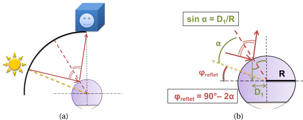
FIGURE 2.35 – Vue en coupe - Rayons et angles associés de la méthode en demi-sphère.
