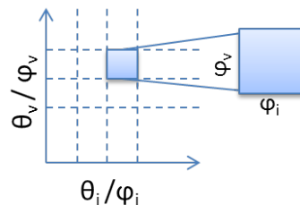
FIGURE 2.39 – Espace de représentation initiale des données de BRDF complète.
