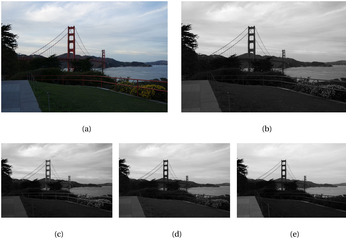
FIGURE 2.12 – L'espace couleur RGB - Composition et décomposition.
