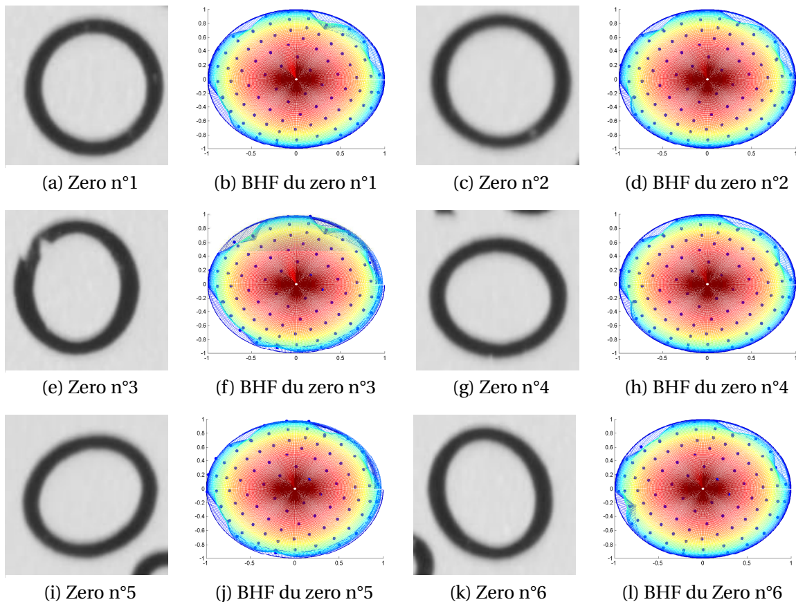
FIGURE 4.23 – Cas réels et représentations associées des BHF de l'homogénéité dans le plan de référence X-Y.
