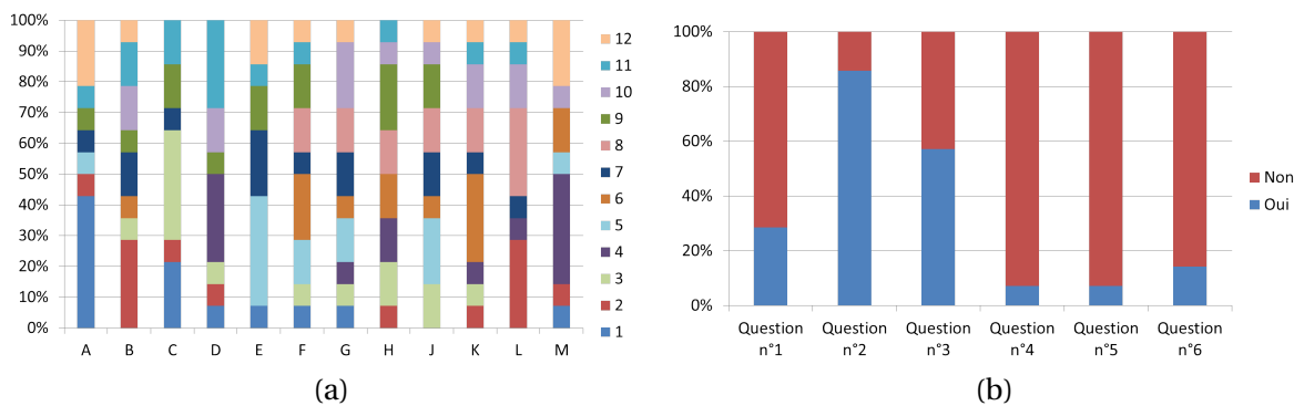
FIGURE 3.25 – Distributions des réponses pour les deux tests à partir de personnes averties à la définition de hiérarchie d’anomalies fines.
