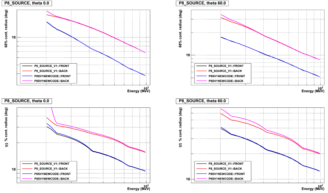
FIGURE 4.3 – Illustration des performances de la PSF pour les deux définitions de la déviation angulaire. Colonne de gauche : pour des événements à incidence normale ( \theta=0^\circ ). Colonne de droite pour des événements hors axe ( \theta=60^\circ ). Pour les deux colonnes, en haut : confinement à 68%, en bas à 95%. On observe que l'écart le plus notable apparaît pour le confinement à 95% dans le cas d'événements de basse énergie, hors axe qui se sont convertis dans le fond du trajectographe. Figure réalisée à l'aide de prototypes d'IRF Pass 8 (P8SOURCE_V1).
