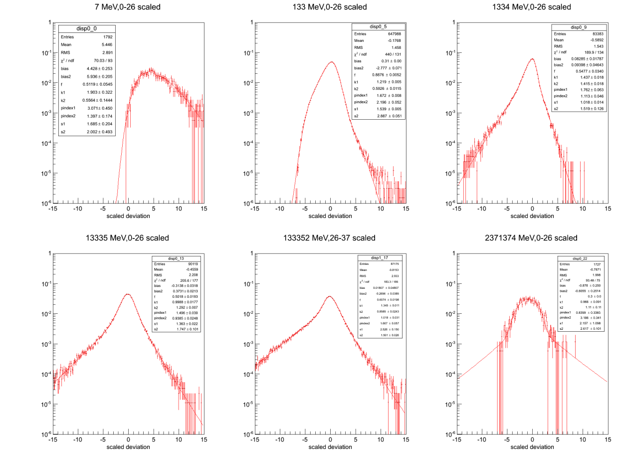
FIGURE 4.20 – Variation de la forme de l’histogramme de la dispersion en énergie en fonction de l’énergie pour des événements SOURCE : :FRONT situés dans des bins d’énergie moyenne (de droite à gauche et de haut en bas), 7 MeV, 133 MeV, 1 GeV, 13 GeV, 133 GeV et 2 TeV, et ayant un angle d’incidence entre 0 degré et 26 degrés (incidence normale). On voit que la nouvelle paramétrisation de la dispersion en énergie parvient à s’ajuster convenablement sur toute la gamme d’énergie du LAT soit 6 ordres de grandeur.
