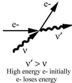
FIGURE 1.2 – Vue schématique du processus de diffusion Compton inverse d'un électron sur un photon d'énergie E = h\nu , produisant un photon d'énergie E' = h\nu' supérieure à E , ayant pour conséquence une perte d'énergie de l'électron.
