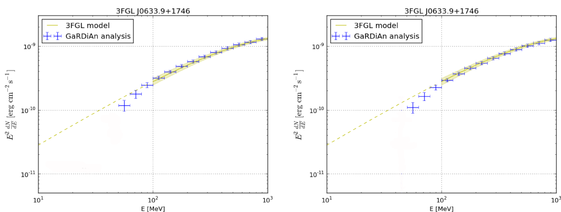
FIGURE 6.19 – SED du pulsar Geminga obtenue à l'issue de l'analyse GaRDiAn (points bleus), à gauche en modélisant la source par une série de lois de puissance d'indice fixe à -2 et à droite avec un indice fixe à -1.
