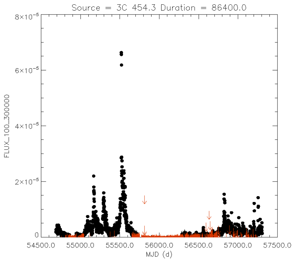
FIGURE 6.15 – Courbe de lumière du blazar 3C454.3 mesuré par le LAT. Chaque bin représente 1 jour de données. On remarque une baisse significative d'activité entre 2012(MJD~56000) et 2014(MJD~56700). Source : http://fermi.gsfc.nasa.gov/ssc/data/access/lat/mslqc/
