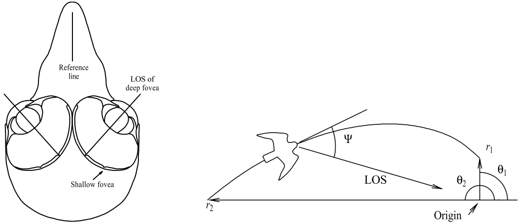
FIGURE 1 – Optimisation de la trajectoire chez les faucons pèlerins. Fig. (a) : structure anatomique de l’œil du faucon avec la fovéa (la zone spécialisée dans la vision aiguë) visant à environ 45 degrés par rapport à l’axe frontal, image prise de [Tuc00]. Fig. (b) : trajectoire en spirale suivie par le faucon afin d’optimiser la perception visuelle et l’aérodynamique pendant le vol vers sa proie, image prise de [TTAE00].
