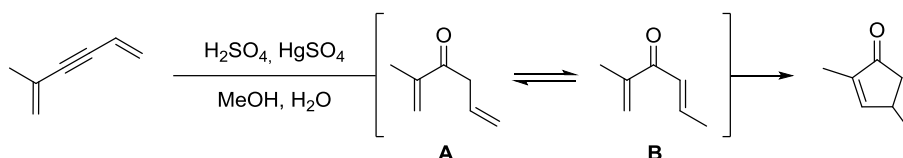
Schéma 34. Hydratation et cyclisation de diényne
