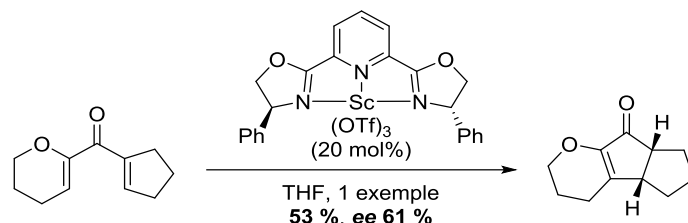
Schéma 83. Première version asymétrique de la réaction de Nazarov, Sc(III)-pyBOX
