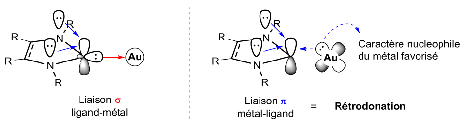
Schéma 17. Liaison Au(I)-NHC
