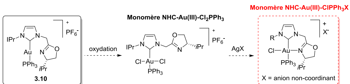
Schéma 132. Vers des catalyseurs chiraux d'or(III) NHC-oxazoline-phosphine
