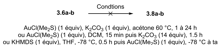
Schéma 115. Synthèse directe des complexes Au(I)
