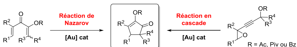
Schéma 72. Un produit, deux voies de synthèse
