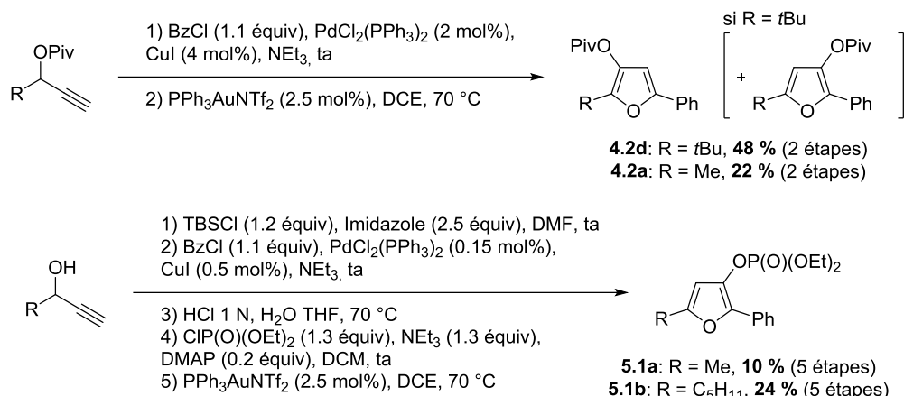
Schéma 158. Synthèses de furanes trisubstitués
