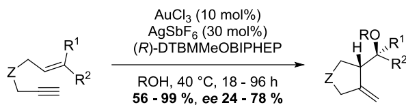
Schéma 108. Alkoxycyclisation, Au(III) vs Au(I)
