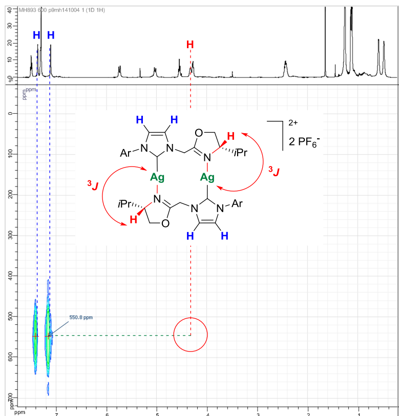
Schéma 122. Visualisation de la coordination oxazoline-métal en RMN 107/109 Ag
