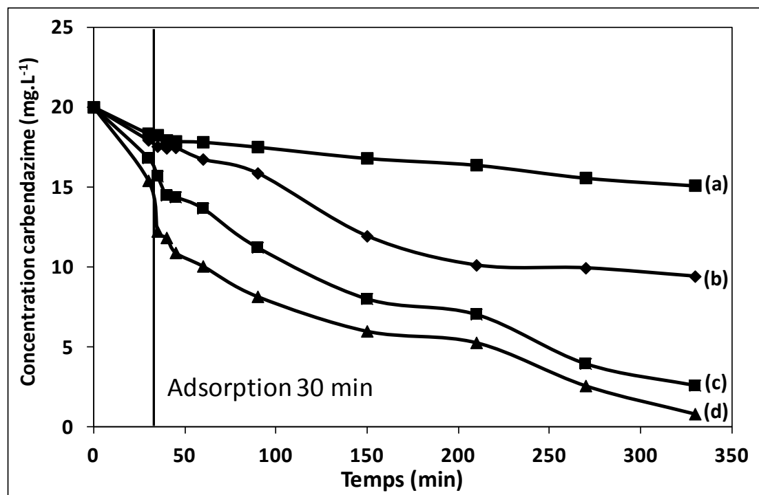
Figure IV-19- Courbes cinétiques des réactions de décomposition du carbendazime sur la série des catalyseurs préparés sur la silice SiO 2 (0.3M+MA) (a) Fe(6)/Ni(6)_SiO 2 (0.3M+MA)_CYC_Cl, (b) Fe(6)/Co(6)_SiO 2 (0.3M+MA)_CYC_Cl, (c) Fe(6)/Zn(6)_SiO 2 (0.3M+MA)_CYC_NO 3 et (d) Fe(6)/Cd_SiO 2 (0.3M)_CYC_NO 3
