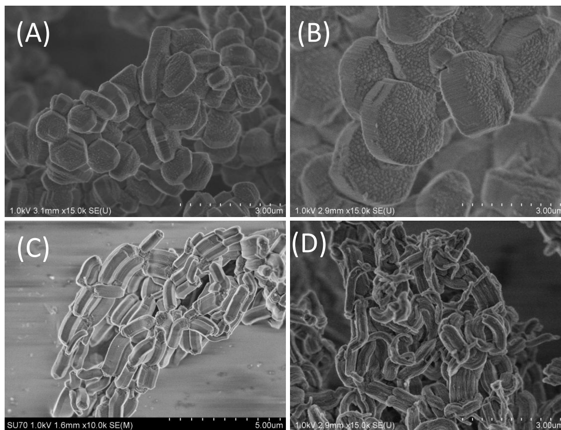
Figure I-12- Des micrographies MEB obtenues sur les trois silices (A) \text{SiO}_2 (0.3M), (B) \text{SiO}_2 (0.3M+MA) et (C) et (D) \text{SiO}_2 (2M) traitées hydrothermalement à 130^\circ\text{C} , 33 heures et calcinées
