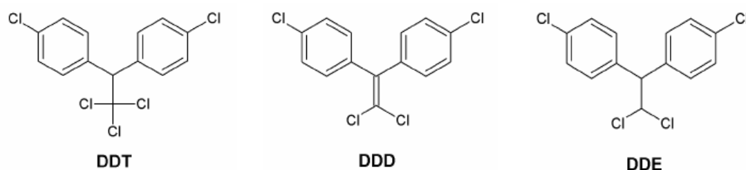
Figures IV-1- Formules moléculaires des molécules DDT, DDD et DDE. Interdits en Europe.
