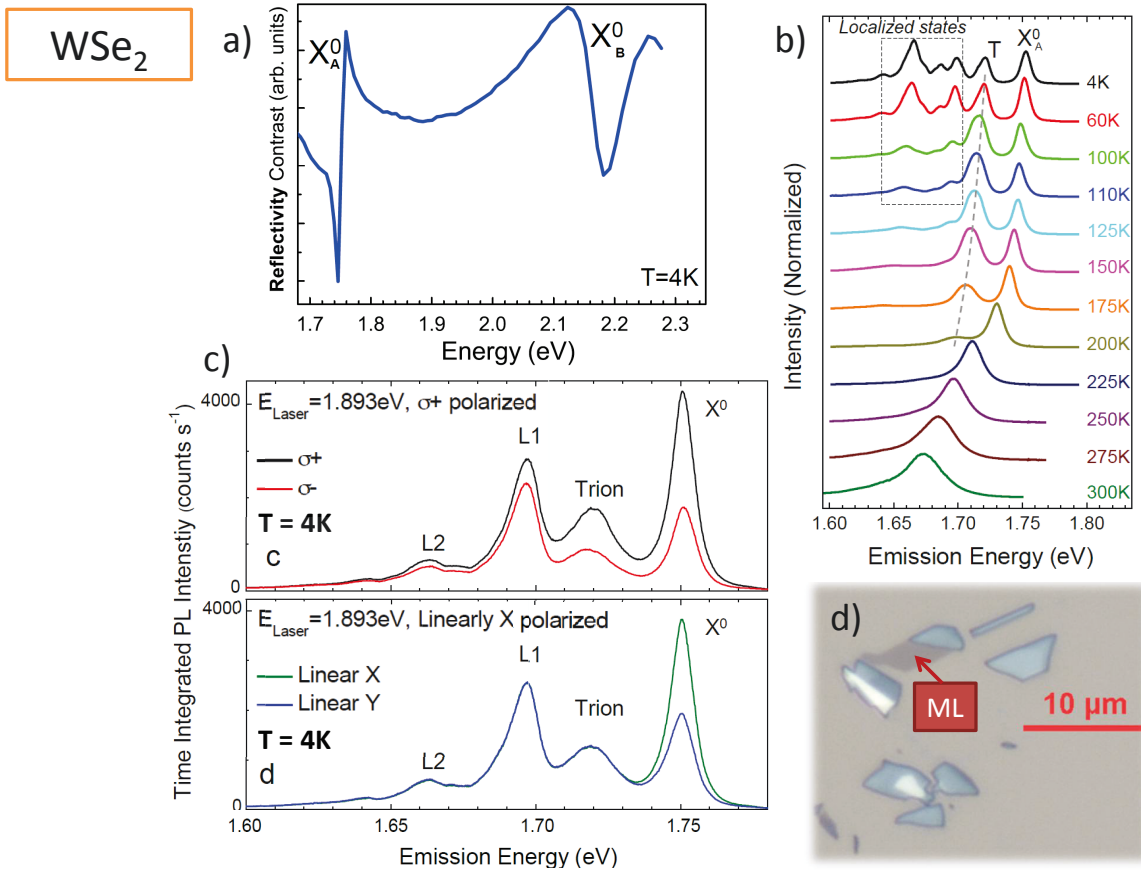
Figure 5: Vue d'ensemble de l'échantillon : monocouche de \text{WSe}_2 (a) Mesure de réflectivité permettant d'extraire un écart en énergie entre les transitions X_A^0 et X_B^0 d'approximativement \approx 450 meV, in good agreement with both experimental and theoretical values of the literature [26] (b) Dépendance en température de l'émission de photoluminescence (c) Polarisation circulaire et linéaire de la photoluminescence sous excitation respectivement circulairement et linéairement polarisée (d) Image du cristal monocouche observé au microscope optique
