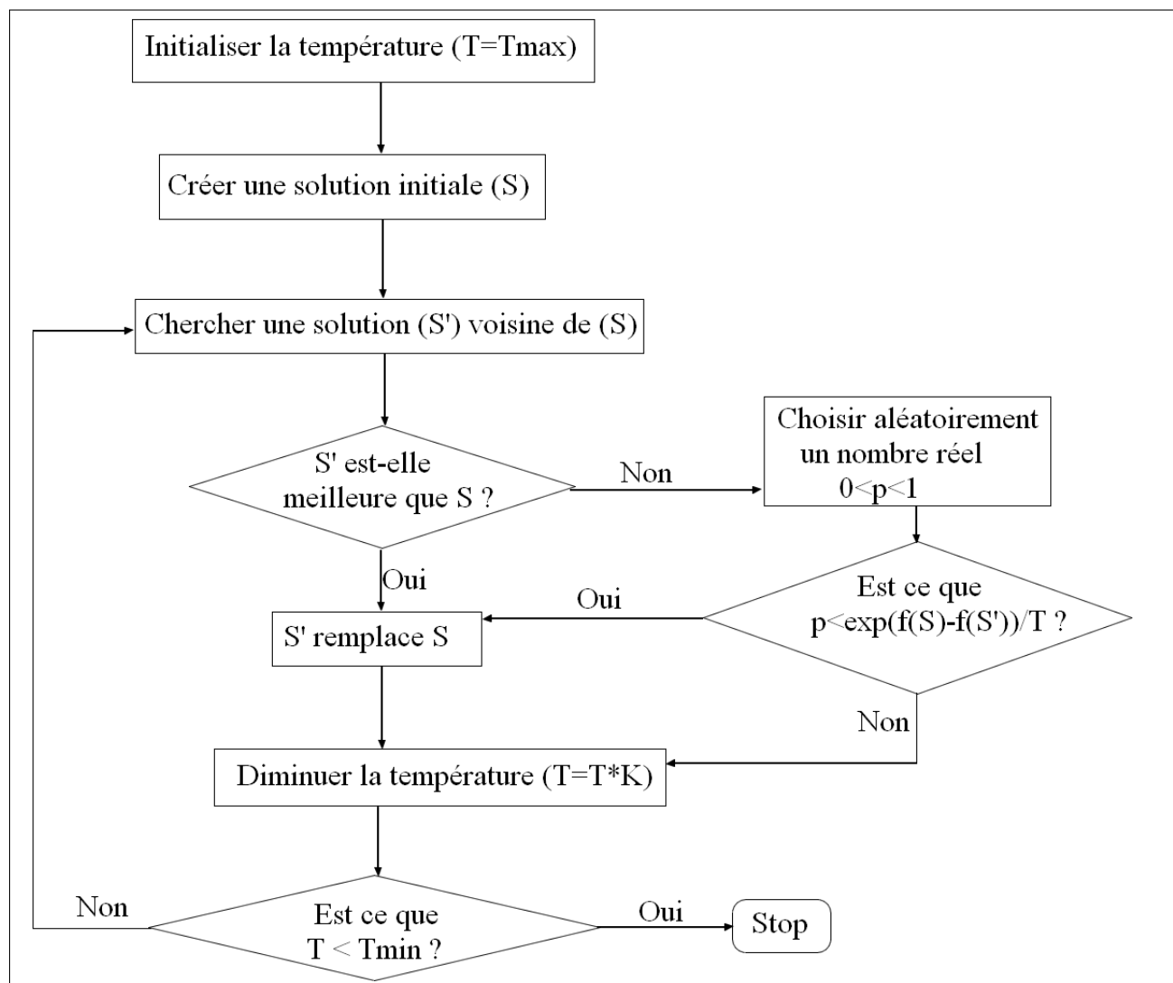
FIGURE 44 – Algorithme du recuit simulé
