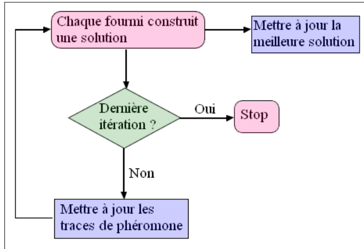
FIGURE 40 – Algorithme de colonie de fourmis
