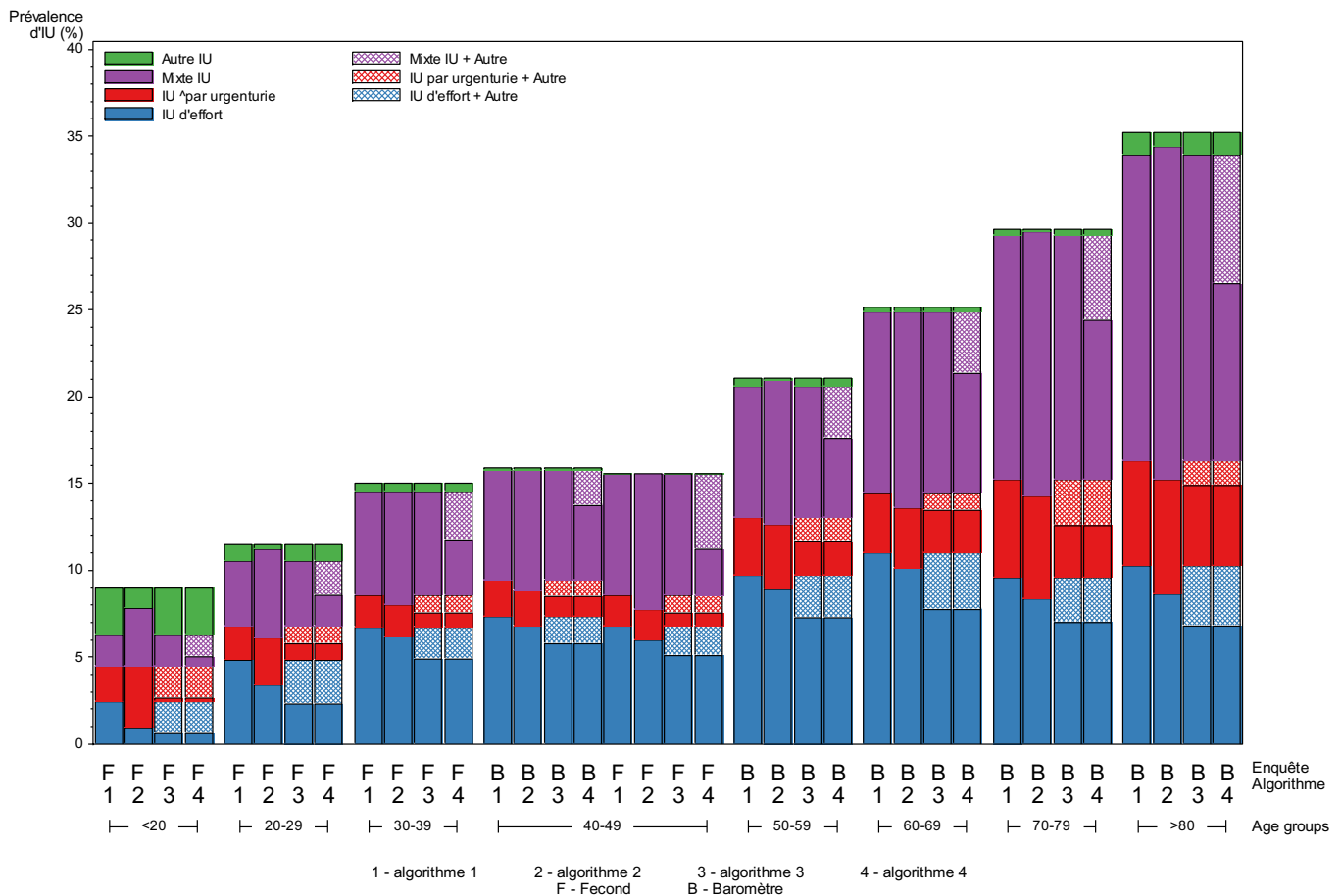
Figure 3.5. Distribution des types d'UI dans le Baromètre (B) et Fecond (F) avec les 4 algorithmes retenus
