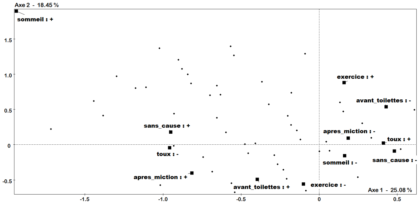
Figure 3.10. Analyse des correspondances multiples (ACM) montrant les projections des 6 circonstances (sans la circonstance ‘tout le temps’) identifiées de fuites urinaires (variables actives dans les carrés noirs) dans les données de Fecond sur l’axe 1 et l’axe 2. Les points représentent les individus
