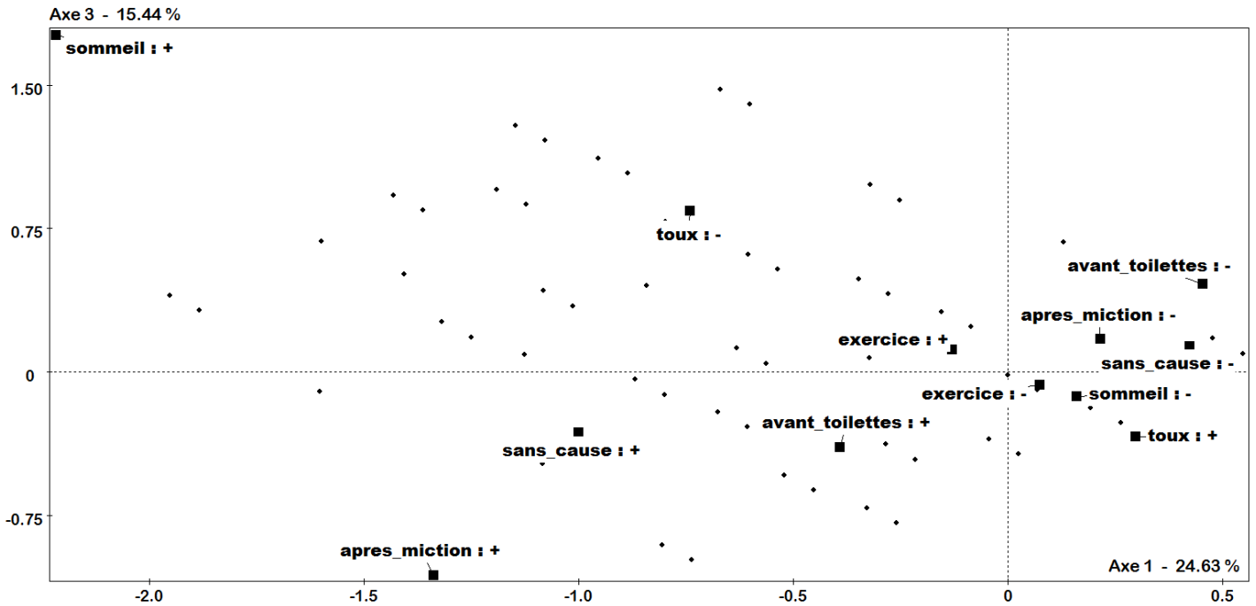
Figure 3.20. Analyse des correspondances multiples (ACM) montrant les projections des 6 circonstances identifiées de fuites urinaires (variables actives dans les carrés noirs) dans les données regroupées sur l'axe 1 et l'axe 3. Les points représentent les individus
