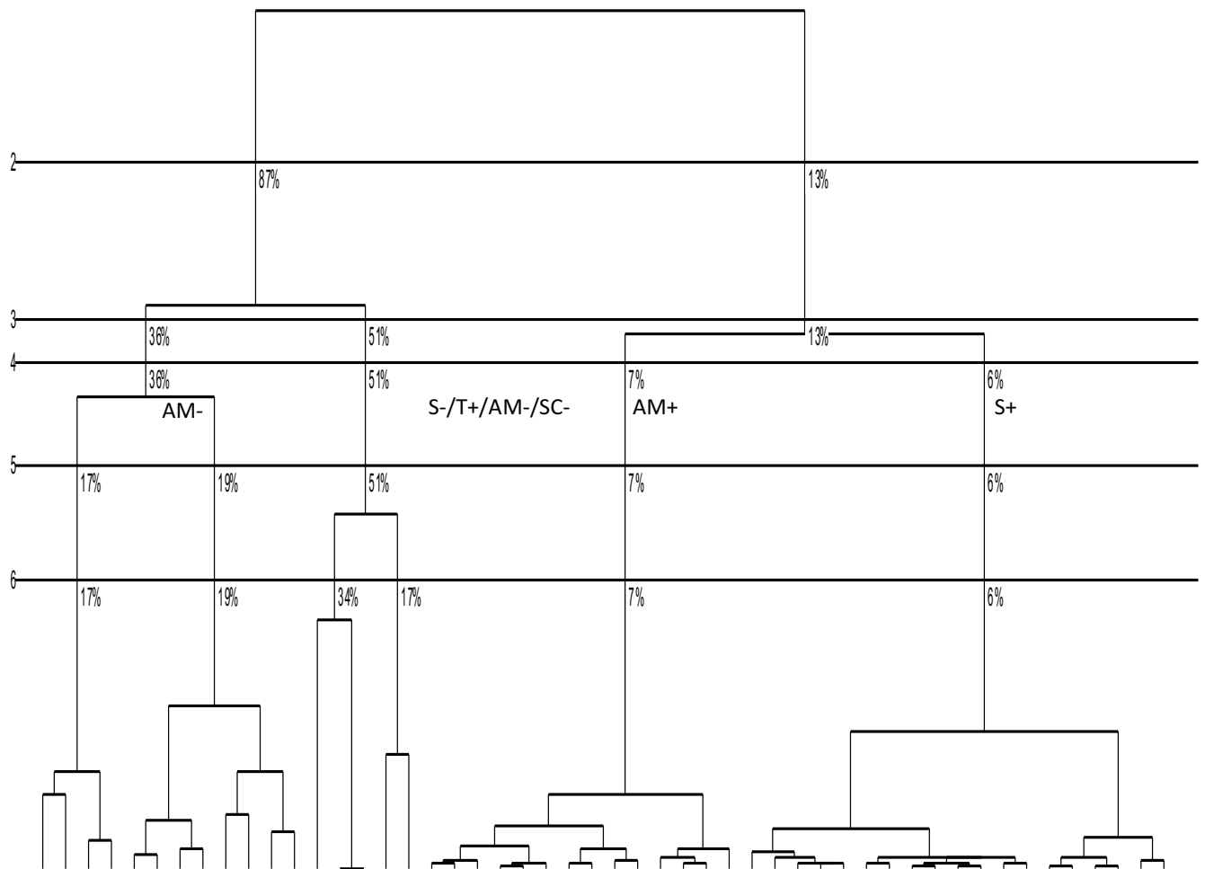
Figure 3.8. Dendrogramme des femmes incontinentes du Baromètre avec 6 circonstances. Les lignes horizontales identifient les niveaux possibles de coupures (S – sommeil, T – toux, AM – après miction, SC – sans cause)
