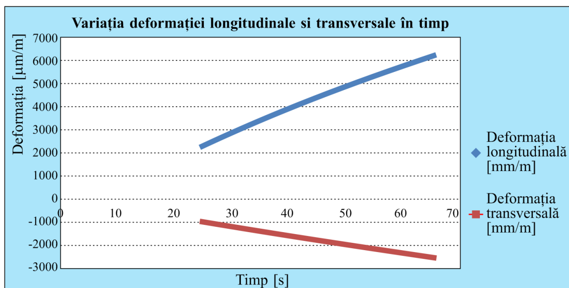
Fig. 5.33. Variația deformației longitudinale și transversale la tracțiune în funcție de timp.
