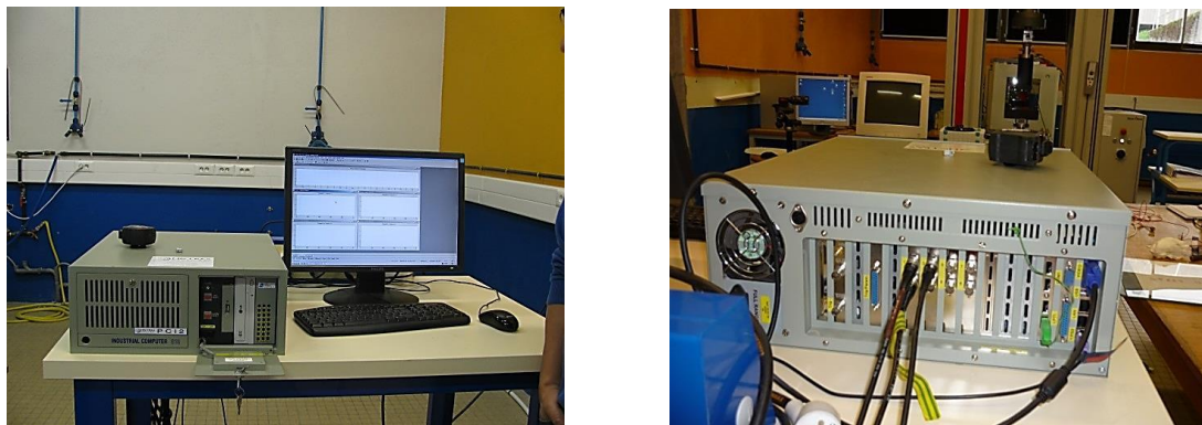
Fig. 5.8. Sistem de detectare a microfisurilor bazat pe metoda emisiei acustice.
