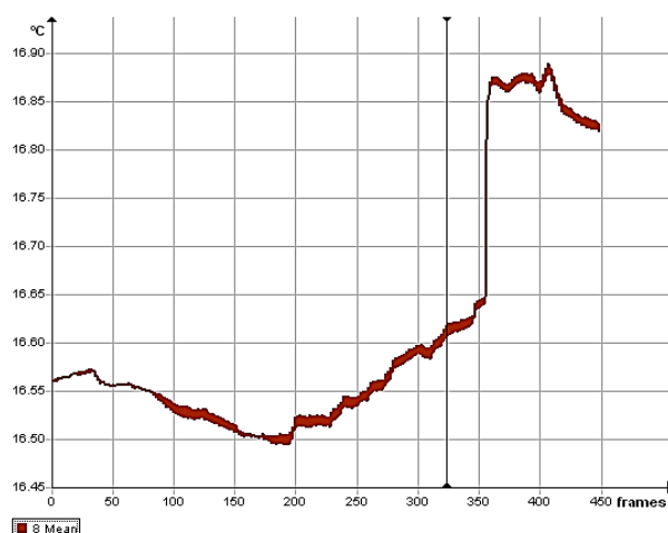
Fig. 5.84. Variația temperaturilor medii în zona de delaminare – etapa finală.
