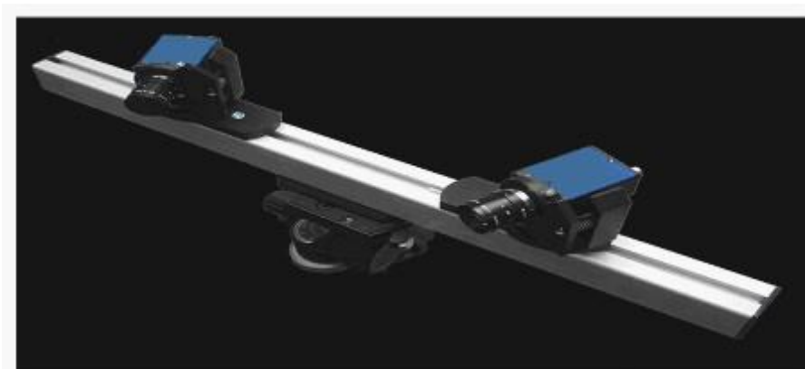
Fig. 2.32. Montaj realizat pentru detectarea defectelor prin metoda corelării imaginilor video, după [Szava et al., 2013].
