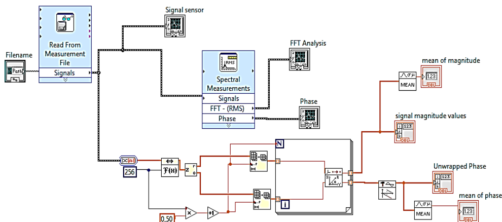
Fig. 5.23. Code du programme LabVIEW DC_3 d'analyse fréquentielle.
