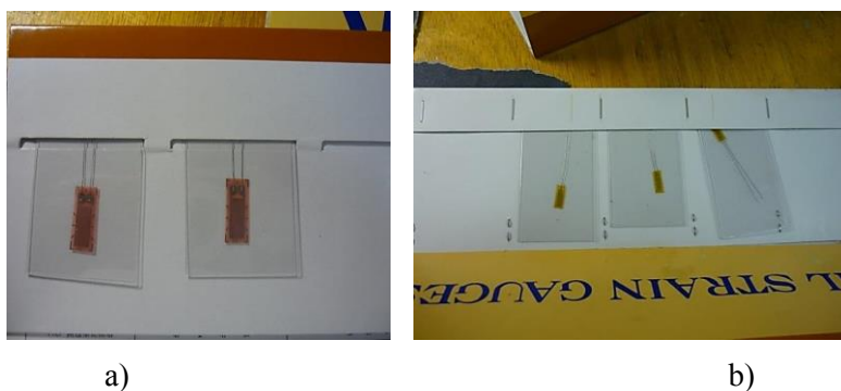
Fig. 5.15 Mărci tensometrice utilizate pentru determinarea deplasărilor în cazul încercării epruvetei la încovoierea în 4 puncte: tip N11 – FA – 8 – 350 – 11 (a); tip N11 – MA – 5 – 120 – 11 (b).
