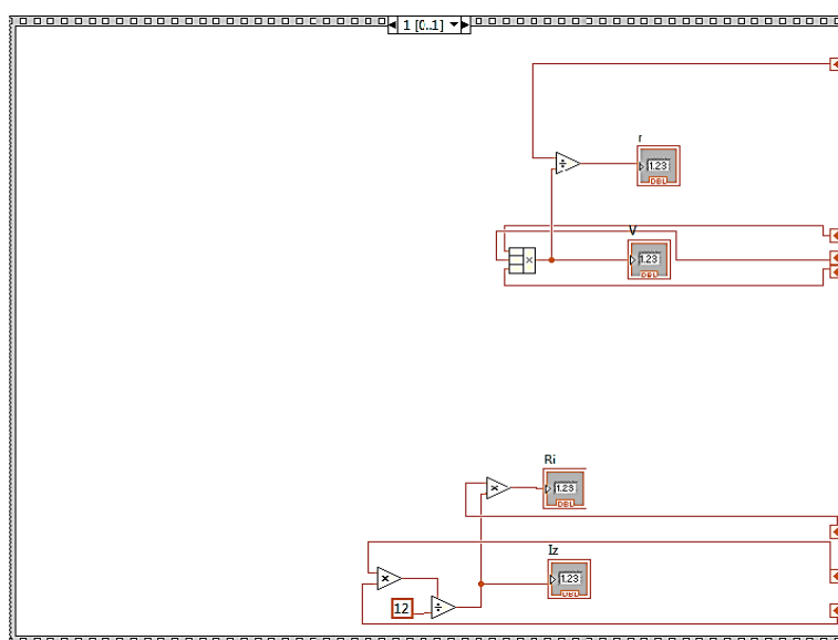
Fig. 5.38. Diagrama aplicației de calcul a variabilelor la încovoiere (cu considerarea pantei) – secvență II (program DC_1).
