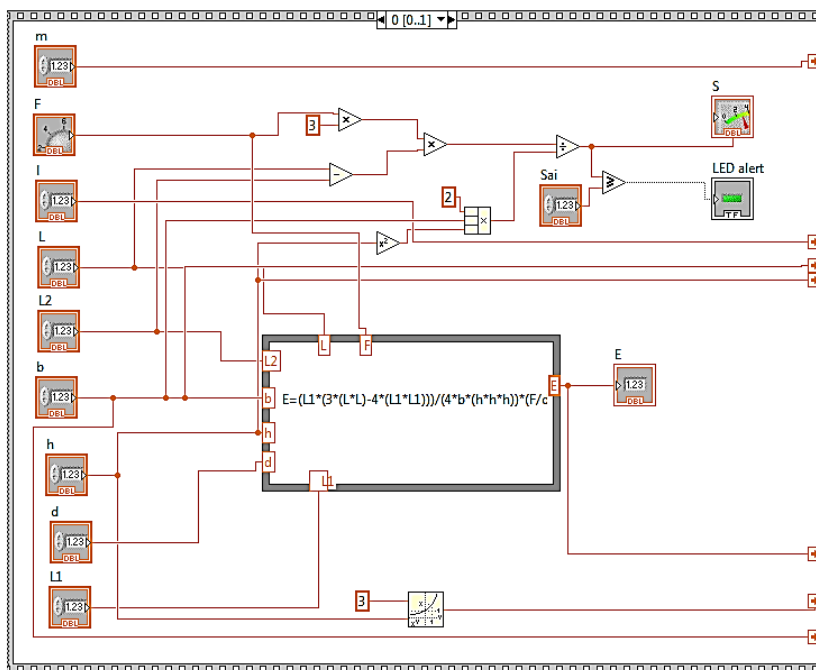
Fig. 5.37. Diagrama aplicației de calcul a variabilelor la încovoiere (cu considerarea pantei) – secvență I (program DC_1).
