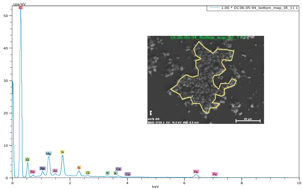
Figure 2-17. Spectre EDX du fragment DC94 écrasé sur la cellule diamant (ø #3_bottom). La zone en jaune sur l'image SE définie la zone sur laquelle a été enregistré ce spectre.
