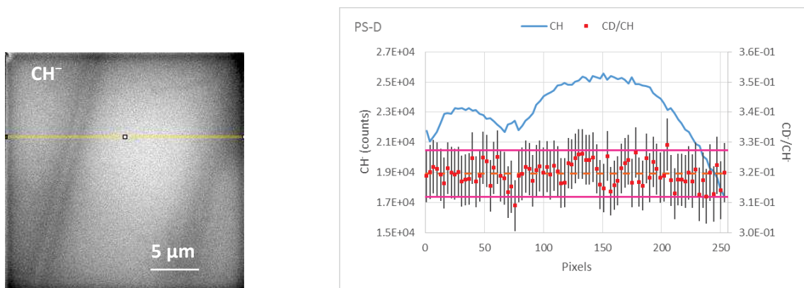
Figure 4-11. Sur la gauche, l'image balayée de CH^- (de taille 25 \times 25 \mu m^2 ) sur PS-D sommée sur 100 trames (de 40 à 139) lorsque le plateau de la Figure 4-7 est atteint, avec un profil de ligne horizontale (ligne en jaune sur l'image) de 3 pixels de largeur. Sur la droite, les évolutions du nombre de coups en ions CH^- et du rapport CD^-/CH^- , le long du profil tous les 3 pixels. Les barres d'erreur (en noir) sont en 2\sigma . La valeur moyenne est calculée sur le plateau et représentée en une ligne orange en pointillés. Les lignes roses représentent l'écart-type expérimental en 2\sigma .
