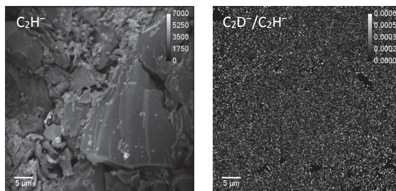
Figure 4-12. Image sommée sur 50 trames de l'espèce C_2H^- (en coups) à gauche et image du rapport C_2D^-/C_2H^- à droite, sur une zone de DonH8 (zone#1). Images de taille 50 \times 50 \mu m^2 , acquises en Juillet 2013 et traitées avec ImageJ. L'image du rapport est lissée et a été seuillée à 10% du maximum sur l'espèce C_2H^- .
