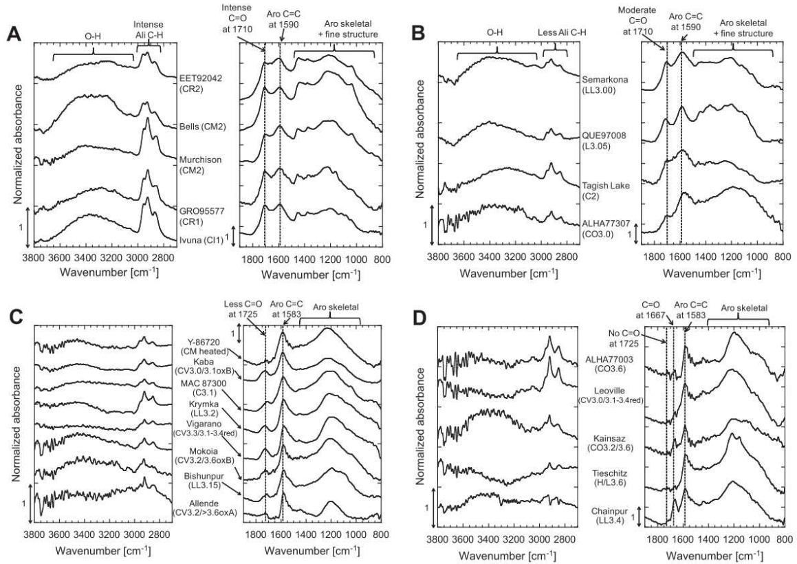
Figure 2-42. Spectres en \mu -FTIR de l'IOM chondritique pour les régions 2800\text{-}2700\text{ cm}^{-1} et 1900\text{-}800\text{ cm}^{-1} . Quatre groupes (A – D) sont représentés, basés sur des caractéristiques spectrales communes. Figure extraite de (Kebukawa et al. 2011).
