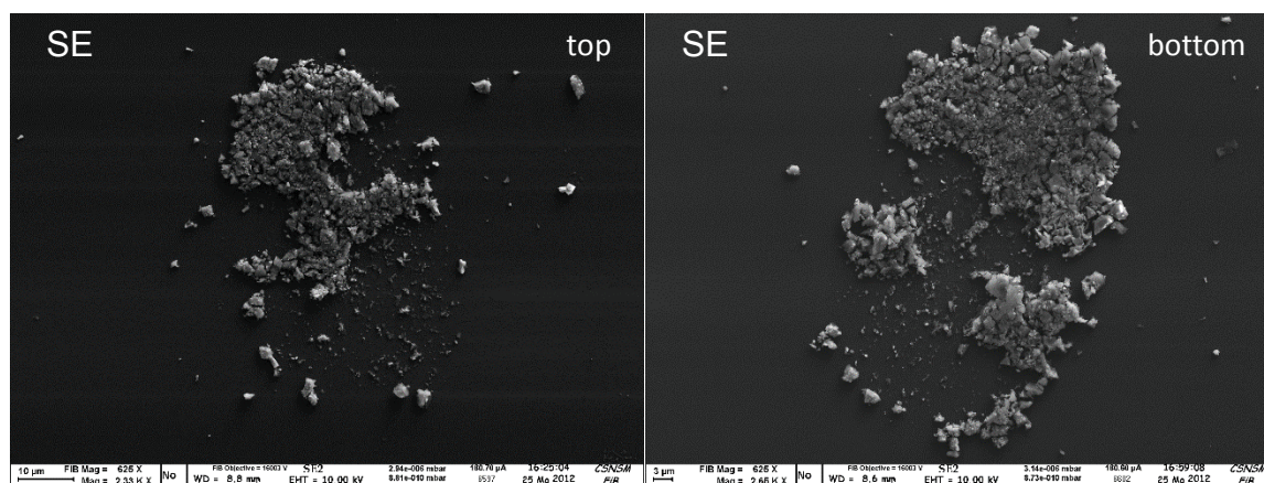
Figure 2-31. Images en SE du fragment de la particule DC19 monté sur la cellule diamant (#15). À gauche, la partie top de la cellule et à gauche la partie bottom de la cellule.
