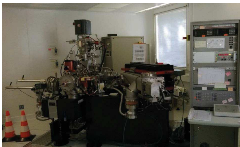
Figure 3-1. Le NanoSIMS-50 au LMI de l'Institut Curie d'Orsay.
