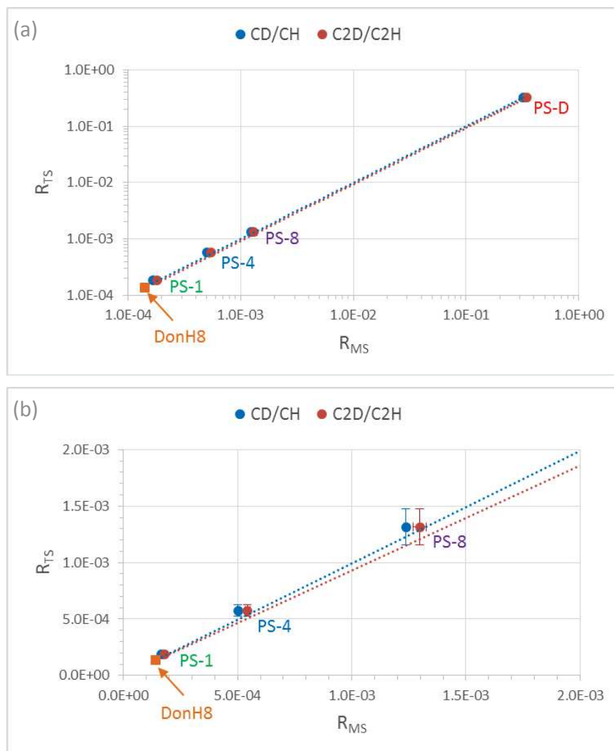
Figure 4-13. Les courbes de l'IMF du rapport CD-/CH- (ligne en pointillés bleue) et du rapport C_2D-/C_2H- (ligne en pointillés rouge) sur l'ensemble de la plage de variation du rapport D/H (a) et fermée sur une partie restreinte de cette plage (b). Les points bleus et rouges font respectivement référence aux rapports CD-/CH- et C_2D-/C_2H- moyens mesurés sur chacun des 4 échantillons. Pour la plupart des points, les incertitudes expérimentales (en 2\sigma ) sont de l'ordre de la taille des points. Les mesures sur l'antracite terrestre (DonH8) sont reportées en un carré orange.
