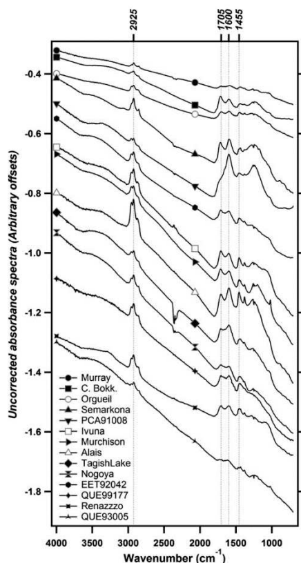
Figure 6-4. Spectres IR de l'IOM de météorites. Figure extraite de (Orthous-Daunay et al. 2013).
