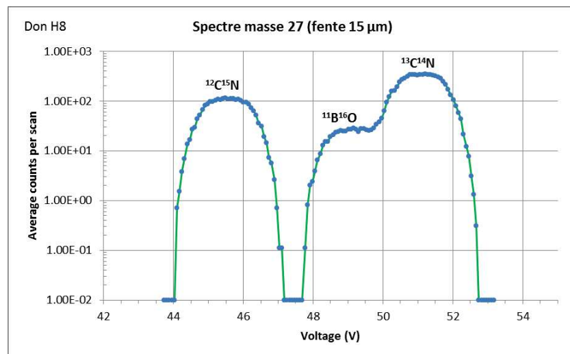
Figure 4-15. Spectres en masse enregistrés à Curie en Juillet 2013 aux masses A = 26 (sur 10 passages), à gauche, et A = 27 (sur 10 passages), à droite, sur DonH8. Voltage step : 0.15 V ; Counting time : 0.54 s.
