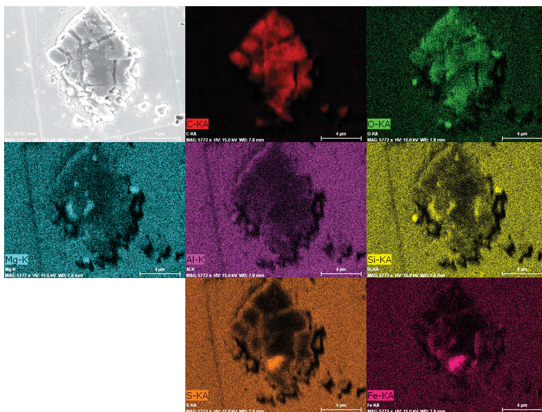
Figure 2-34. Image SE en haut à gauche et cartes EDX de C, O, Mg, Al, Si, S et Fe du fragment de DC119 écrasé sur la lame d'or LO_08-02.
