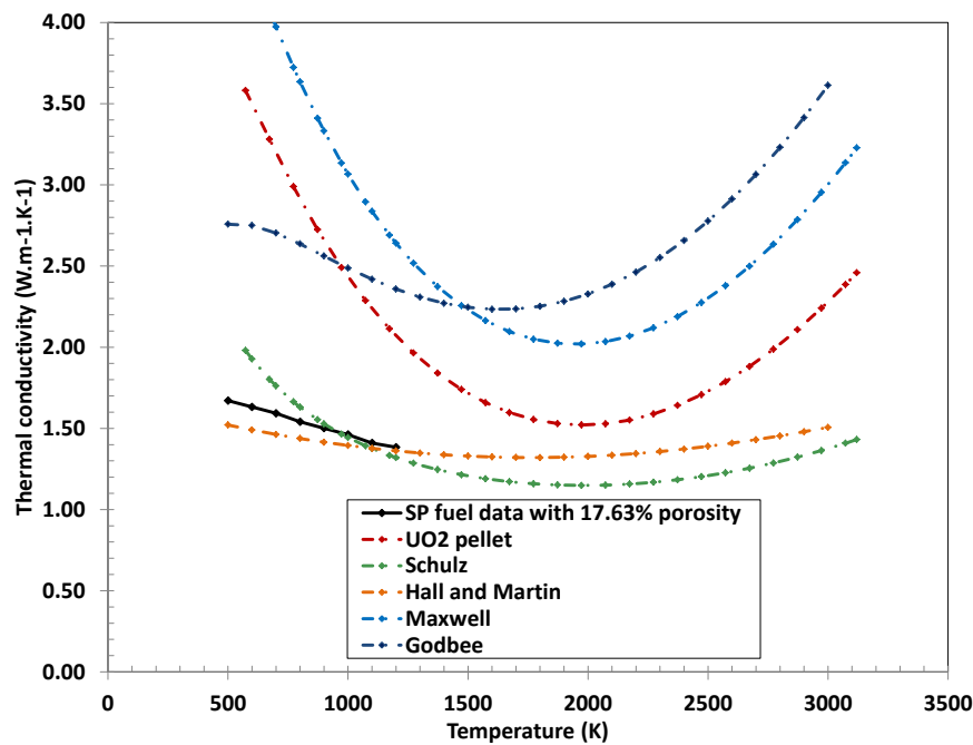
Figure L-4. Conductivité thermique de combustible sphere-pac (SP) \text{UO}_2 (2 fractions de sphères de 1200 \mu\text{m} et 35 \mu\text{m} en diamètre, 0% de striction, 1 bar de pression d'Hélium) pour différentes corrélations et comparaison avec les données tirées de [181].
