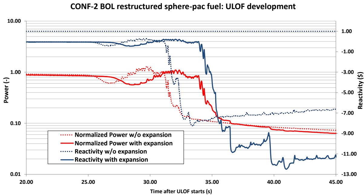
Figure L-16. Evolution de puissance et de réactivité durant un accident de perte de débit primaire dans le cœur CONF2 en début de vie, contenant du combustible restructuré avec ou sans la prise en compte des contre-réactions provenant de la dilatation thermique du cœur.
