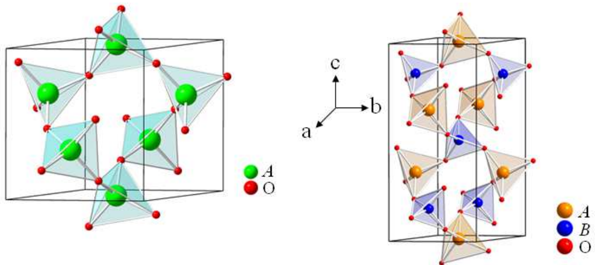
Figure 1.1 : Structure cristalline des homéotypes du quartz AO_2 et ABO_4
