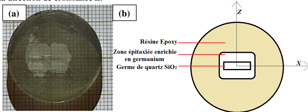
Figure III.8 : Cristal provenant de la croissance \text{SiGe}13 , inclus dans de la résine époxy poli optiquement (a) et schéma explicatif avec les orientations cristallines (b)
