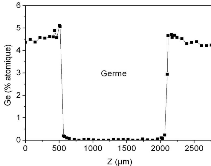
Figure V.18 : Cartographie EPMA de la teneur en germanium dans le cristal issu de la croissance \text{SiGeSn1}
