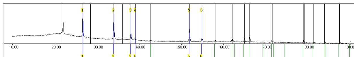
Figure A3.16 : Diffractogramme avec pics de diffraction pointés et pics de diffraction calculés de la phase de type rutile du corps-mère CM SiGeSn 4-4-2 bis
