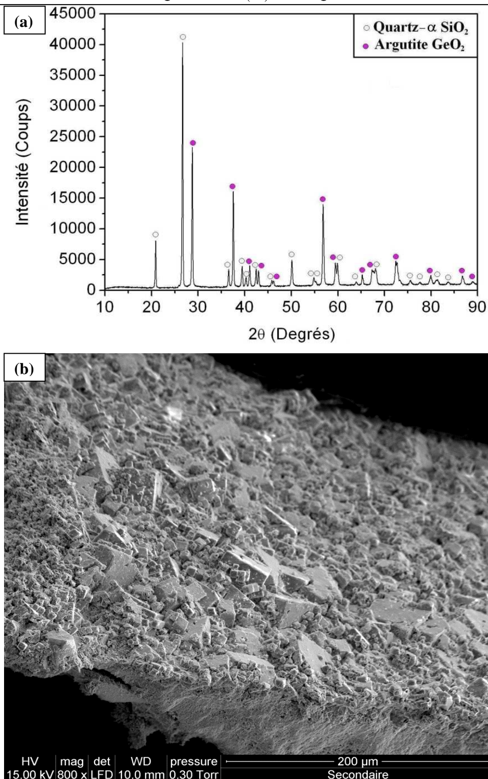
Figure III.10 : Diffractogramme du corps-mère restant après la croissance \text{SiGe}_{12} (a) et son image au MEB avec des électrons secondaires (b)
