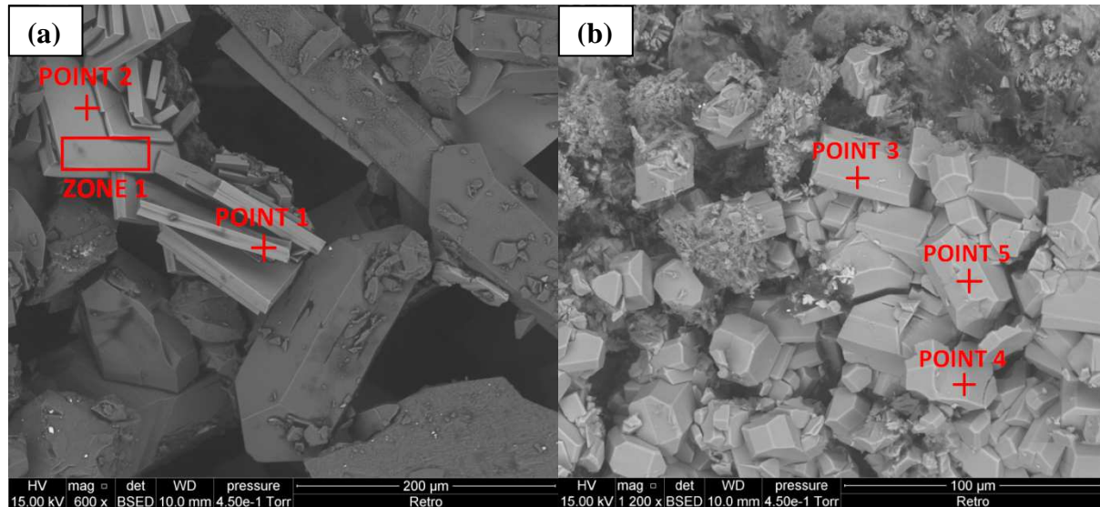
Figure V.12 : Image MEB rétrodiffusée des dépôts cristallins formés en partie haute de l'autoclave durant le cycle de croissance \text{SiSn}_3 (a) et des résidus de corps-mère du cycle de croissance \text{SiSn}_4 (b)
