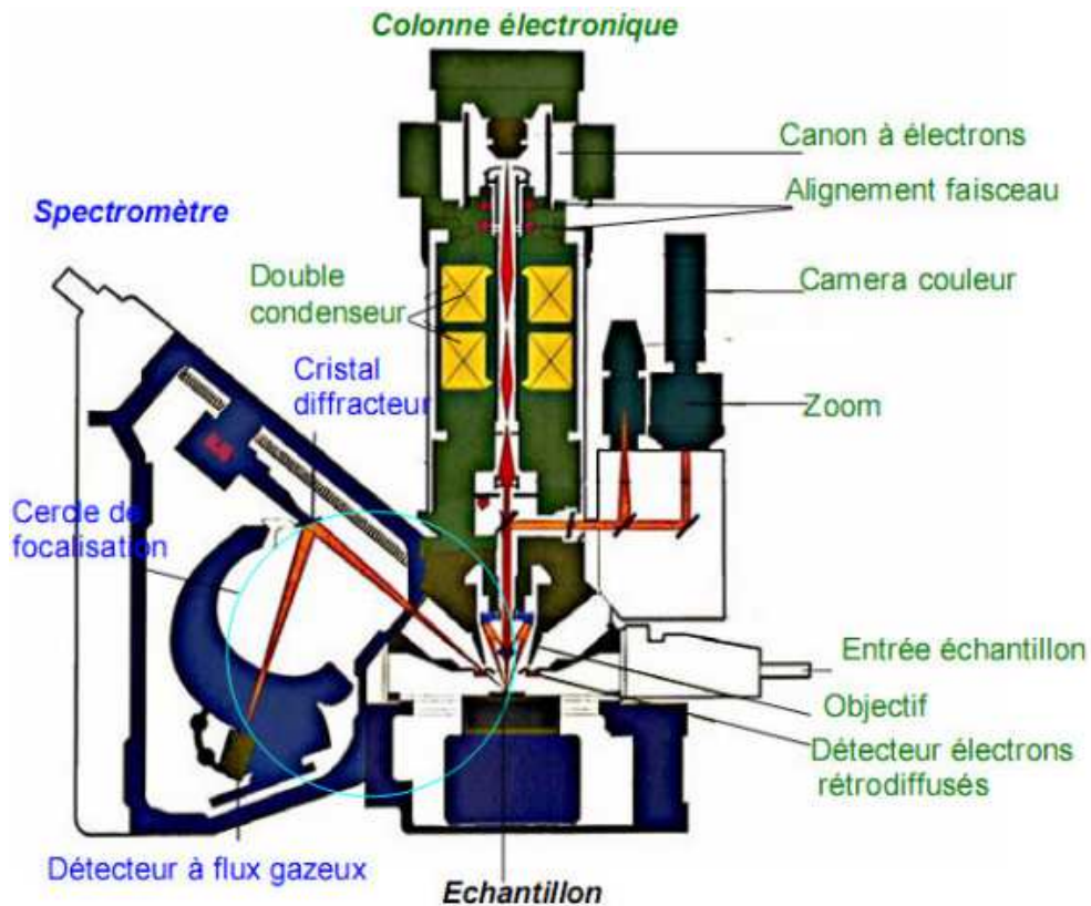
Figure II.25 : Schéma d'une microsconde WDS
