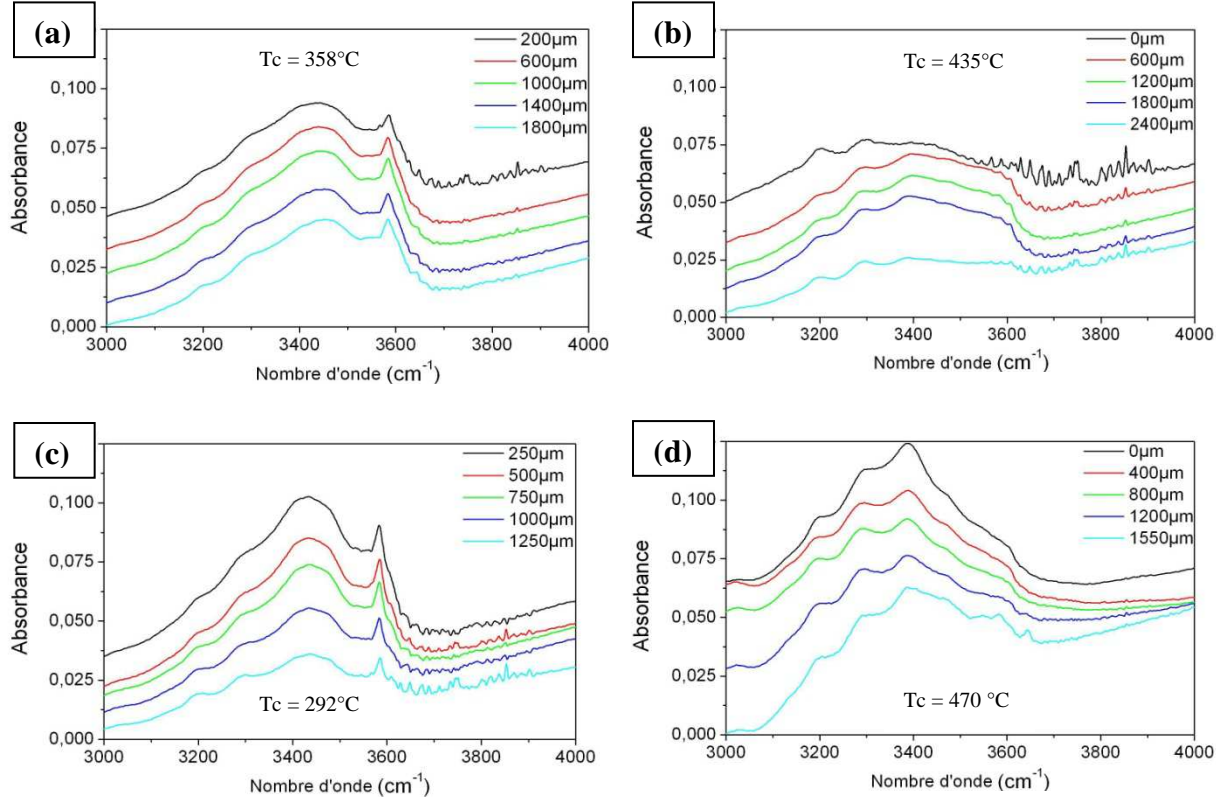
Figure III.16 : Spectres infrarouge des lames SiGe11Y (a) SiGe13Y (b) SiGe14Y (c) et SiGe15Y (d) ces spectres ont été effectués dans la zone épitaxiée du germe (0 \mu\text{m} ) vers le bord du cristal
