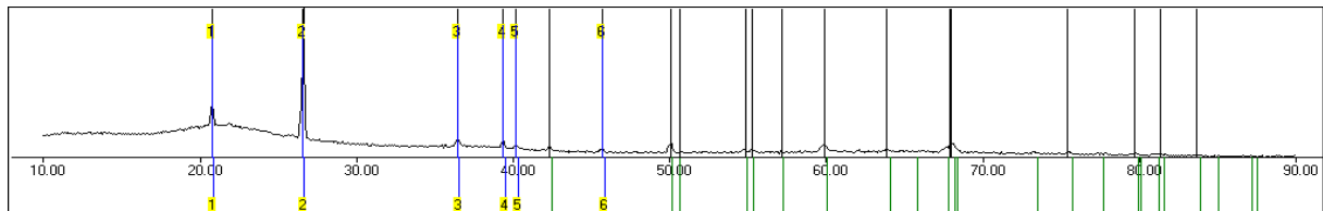
Figure A3.2 : Diffractogramme avec pics de diffraction pointés et pics de diffraction calculés de la phase de type quartz- \alpha du corps-mère VG50B
