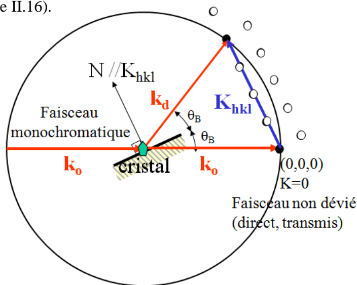
Figure II.16 : Représentation en deux dimensions de la sphère d'Ewald dans le cas d'un rayonnement monochromatique
