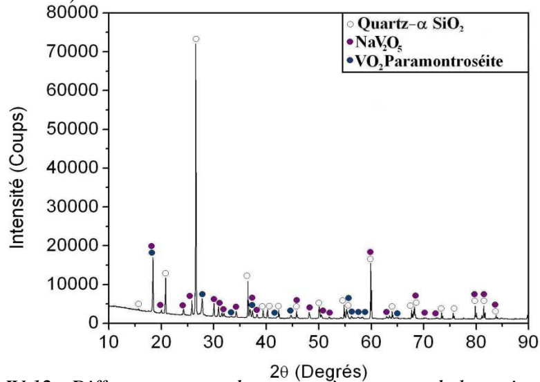
Figure IV.12 : Diffractogramme du corps-mère restant de la croissance SiVI
