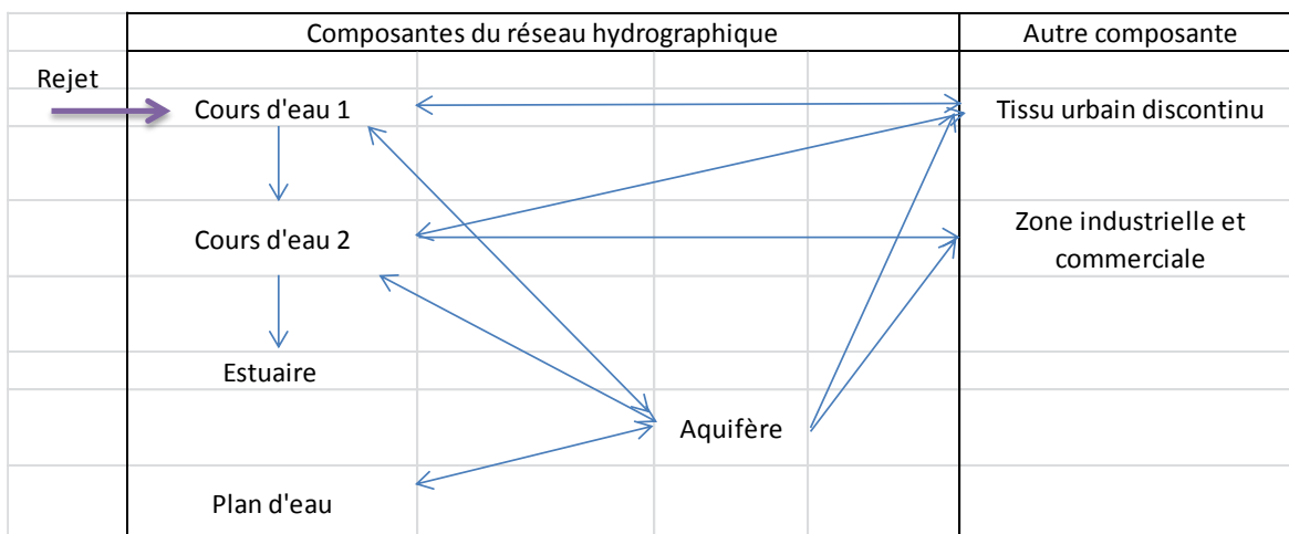
Figure 34: Exemple de diagramme de flux d’eau (flèche violette : indique le milieu dans lequel se fait le rejet ; flèches bleues simples et doubles : indiquent les échanges d’eau entre les composantes du territoire d’étude)
