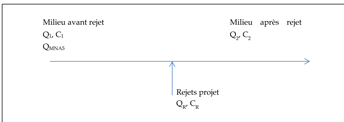
Figure 10 : Schéma pour le calcul de rejet acceptable par un milieu
