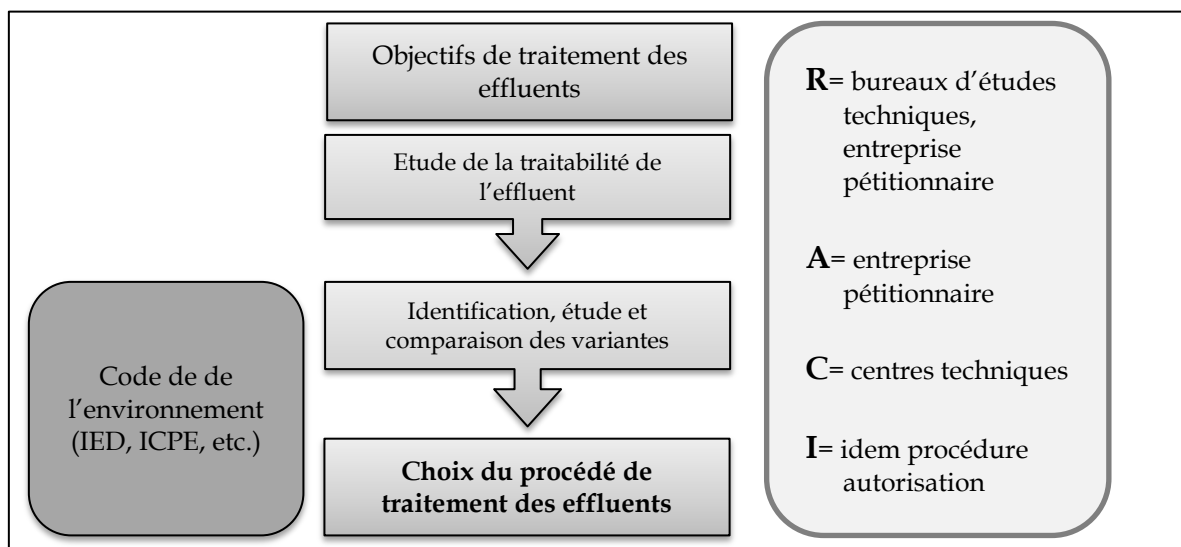
Figure 12 : Schéma du processus de choix du procédé de traitement des effluents
