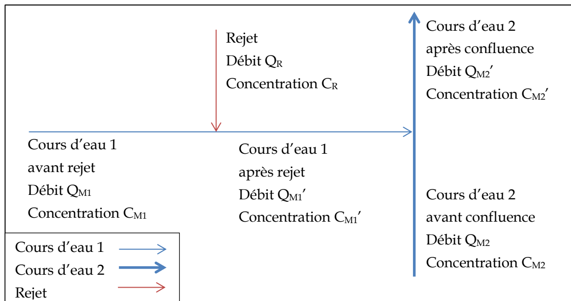
Figure 37 : Exemple de schéma du réseau hydrographique pour le calcul des effets du rejet sur les masses d’eau en aval
