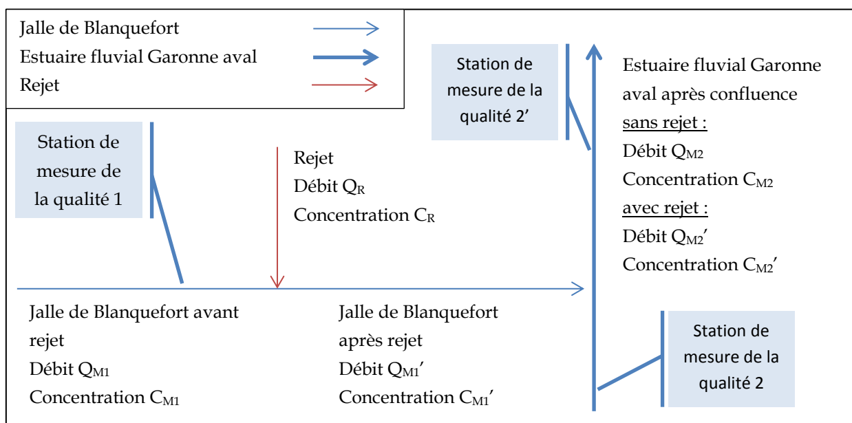
Figure 55 : Représentation du réseau hydrographique local pour le calcul des effets du rejet de l'entreprise Castel Frères (site de Blanquefort) sur les masses d'eau en aval (La Jalle de Blanquefort et l'estuaire fluvial Garonne aval)
