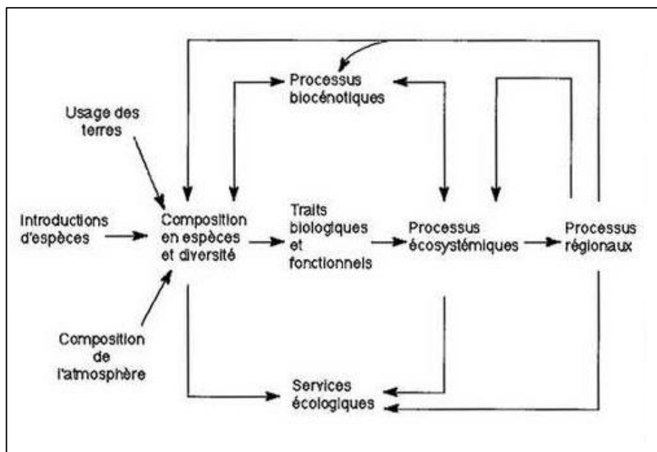
Figure 21 : Relations entre diversité du vivant, processus écosystémiques, services écologiques et facteurs de changement liés aux activités humaines (à gauche) « Ressources biologiques et services écologiques sont l'une des bases essentielles du développement des sociétés humaines qui, mal conduit, pourrait les mener à leur propre déclin. Par processus biocénétiques on regroupe toutes les interactions entre espèces - compétition, prédation, parasitisme, mutualisme. » (Barbault, 2005)
