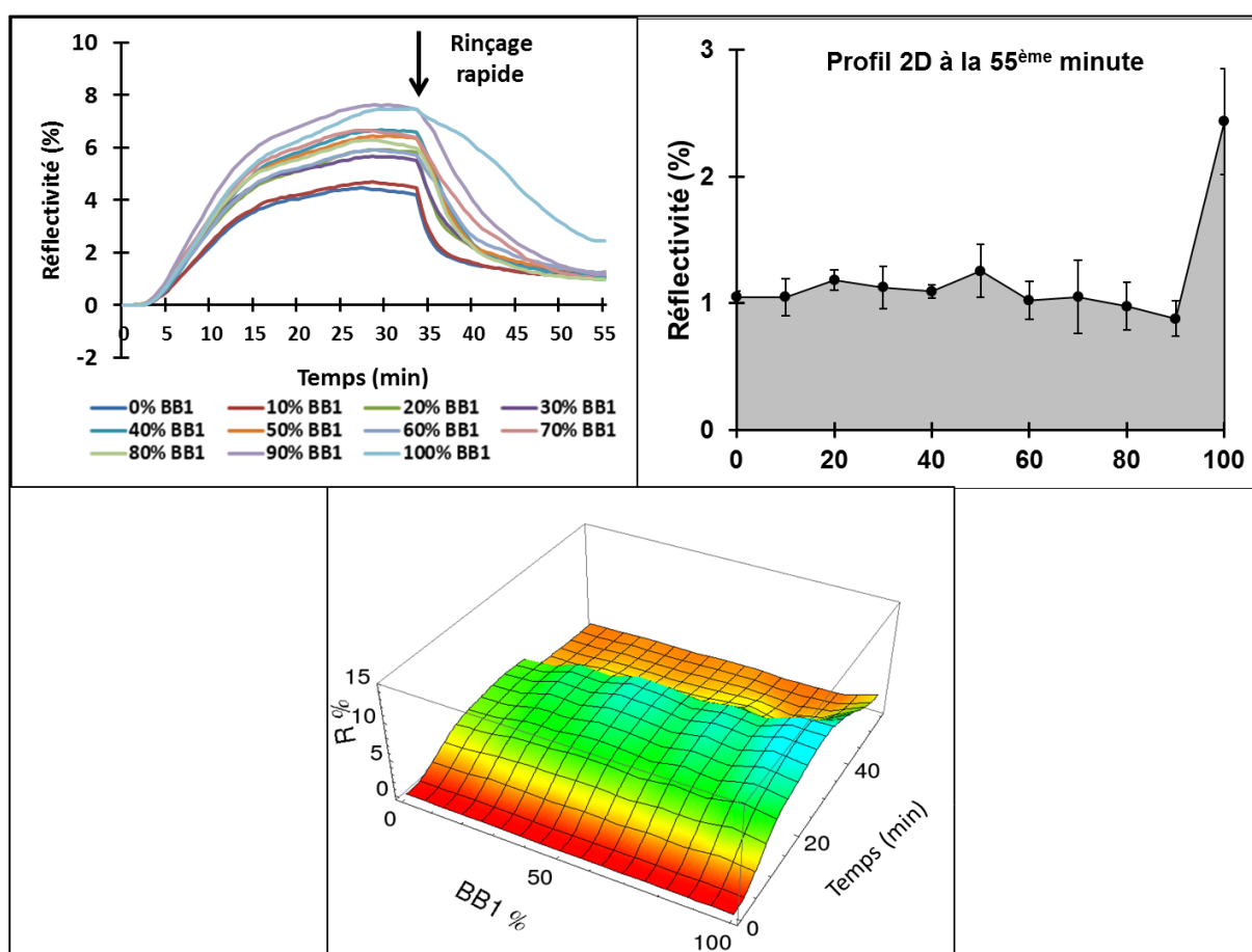
Figure 4-15 : Représentation du sensogramme de la souche E. coli 11775 ainsi que du profil 2D généré à la 55 ème minute soit à la fin de la 2 ème phase de rinçage. L'image 3D obtenue est considérée comme une empreinte de cette souche bactérienne.
