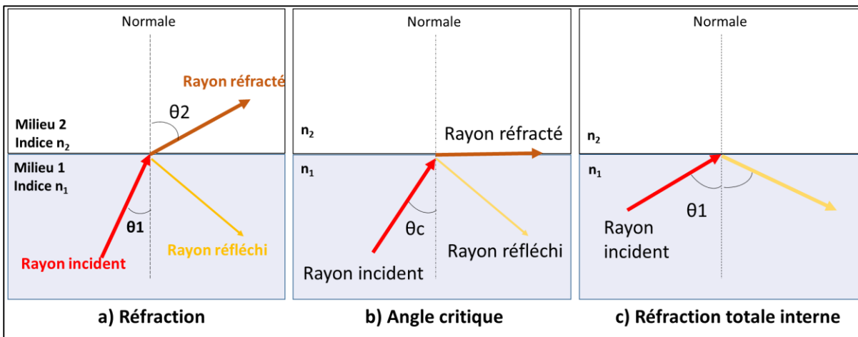
Figure 2-1 : Schéma décrivant la relation de Snell-Descartes ainsi que les rayons réfracté et réfléchi a) Réfraction d'un rayon lumineux pour \theta_1 < \theta_2 , le rayon incident est aussi partiellement réfléchi dans le premier milieu; b) rayon critique lorsque \theta_1 = \theta_c ; et c) réflexion totale interne pour \theta_1 > \theta_c .
