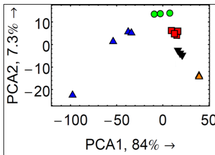
Figure 3-6 : Représentation du résultat d’analyses en composantes principales à partir des images 3D pour les différents échantillons de lait de vache UHT (carré rouge ■) ; lait de vache cru (cercle vert ●), boisson de soja (triangle bleu ▲), boisson de soja chocolat (triangle noir ▼) et de boisson de riz (triangle orange ▲) répétées à 4 reprises.
