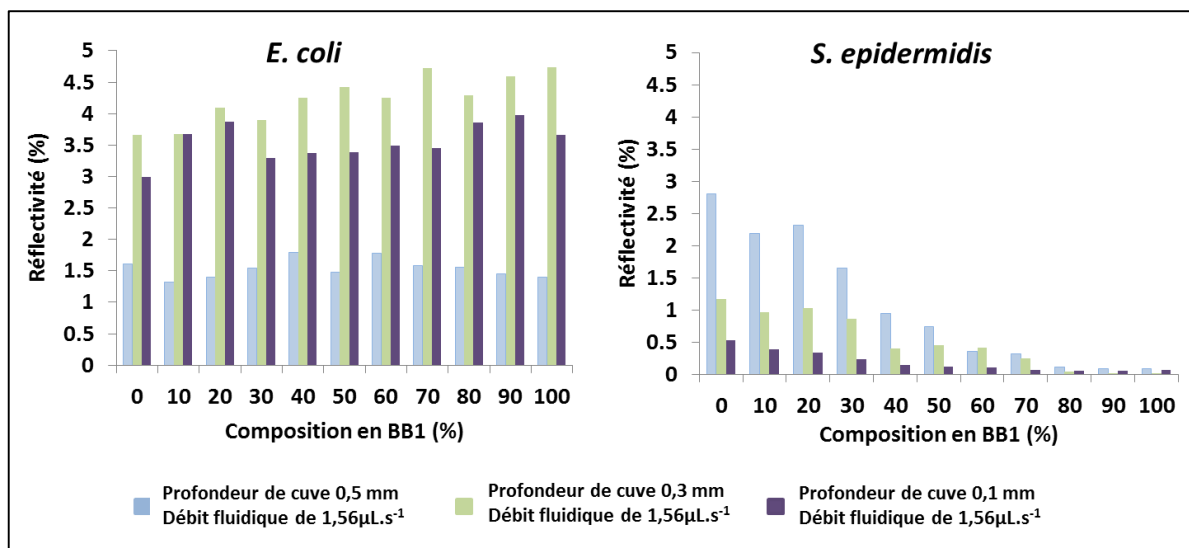
Figure 4-5 : Histogrammes représentant la variation d'intensité mesurée à un débit fluide 1,56 \mu\text{L}\cdot\text{s}^{-1} avec différentes profondeurs de cuves de 0,5 ; 0,3 et 0,1 mm à la fin du r.
