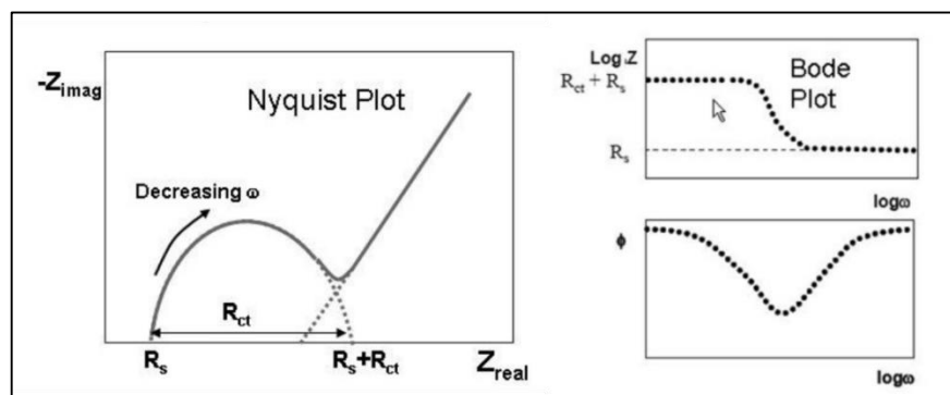
Figure A1-13 : Représentations des diagrammes de Nyquist et de Bode[246]
