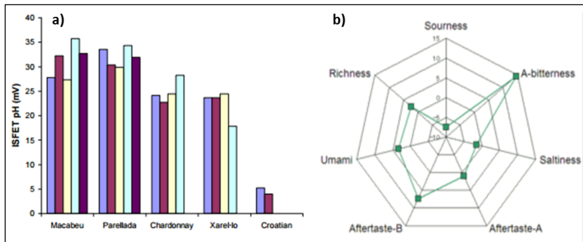
Figure 1-7 : a) Représentation en histogramme d'une analyse de 5 vins par une langue électronique composée de 5 transistor à effet de champ sélectif aux ions (pH ISFET) (parme : Na + , magenta : K + , jaune : Ca 2+ , cyan : Cl - , pourpre : NO 3 - ) [71]. b) Représentation en radar des saveurs décrites par une bière analysée par une langue électronique (capteur de goût) [72].
