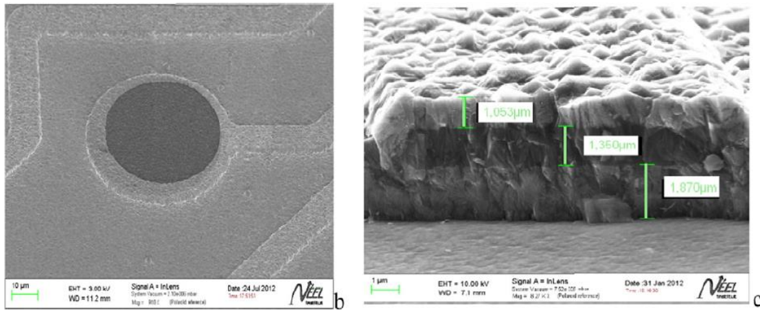
Figure A1-12 : Image MEB d'une microélectrode de diamant et d'une piste clivée verticalement afin d'établir les épaisseurs de films déposés de diamant intrinsèque et de diamant dopé [245].
