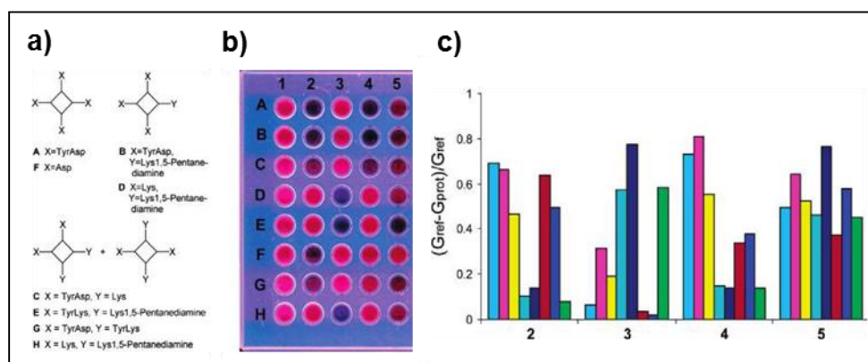
Figure 1-23 : a) Structure schématique des 8 récepteurs porphyriniques notés de A à H b) Fluorescence obtenue après excitation UV à une longueur d'onde de 302 nm. La colonne 1 représente la fluorescence de référence de chacun des 8 récepteurs. Les colonnes 2 ; 3 ; 4 et 5 représentent respectivement les fluorescences obtenues après l'addition des protéines de cytochrome c ; ferrédoxine ; cytochrome c551 et myoglobine à une concentration comprise entre 500 et 600 \mu M. c) Motifs de reconnaissance obtenus pour chacune des protéines lors de l'utilisation des 8 récepteurs de porphyrines. La hauteur des barres quantifie le changement de fluorescence mesurée [125].
