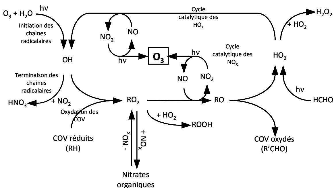
Figure I.3. Représentation schématique des principaux mécanismes impliqués dans la formation d'ozone troposphérique [Camredon et al., 2007]
