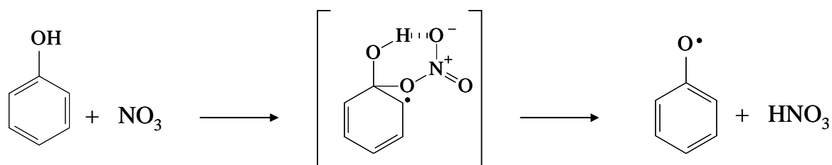
Figure III.22. Mécanisme chimique pour la réaction du phénol avec les radicaux NO 3 [Atkinson et al., 1992].
