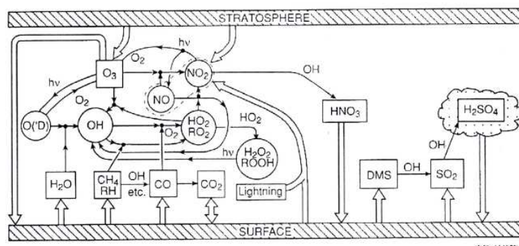
Figure I.2. Diagramme schématisé des processus chimiques et photochimiques clés affectant la composition de la troposphère. Le symbole R correspond à un radical organique et h\nu représente l'absorption du rayonnement solaire [Brasseur et al., 1999].
