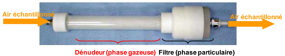
Figure III.2. Photographie d'un dénudeur – filtre.
