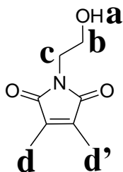
Figure 1 : Structure chimique du 2-hydroxyéthyl diméthylmaléimide.
