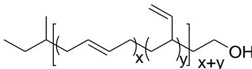
Figure 6 : Structure chimique du polybutadiène monofonctionnel
