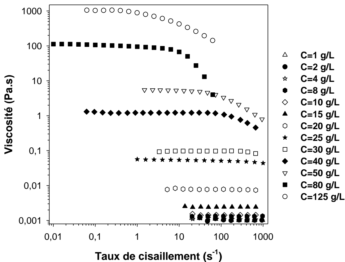
Figure 95: Variation de la viscosité avec le taux de cisaillement pour des solutions de PAME 7 -b-POE 270 -PAME 7 à différentes concentrations.
