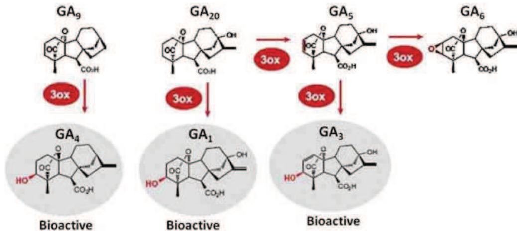
Figure 19: Synthèse des GA bioactives par l'action des GA3-oxydases 3ox = GA3-oxidaeses. (Adapté de Yamaguchi et al., 2008 ; Barker, 2011)
