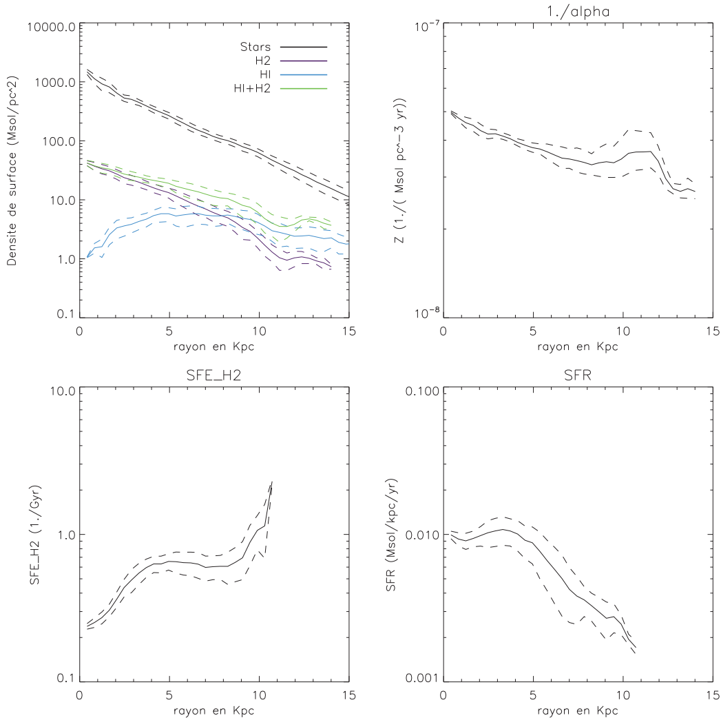
FIGURE 4.2 – Profils radiaux réalisés sur NGC 4501. Haut gauche , les densités de surface de \Sigma_* , \Sigma_{HI} , \Sigma_{H_2} , \Sigma_{HI+H_2} . Haut droite , profil radial de la métallicité Z calculée à partir du "closed box model". Bas gauche , efficacité de formation stellaire. Bas droite , taux de formation stellaire. Les lignes en tirets indiquent l'incertitude liée à la méthode d'extraction des profils radiaux.
