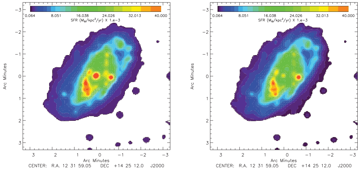
FIGURE 5.3 – Carte de formation stellaire de NGC 4501. Gauche , carte de formation stellaire issue du H\alpha+24 \mu m . Droite , carte de formation stellaire calculée à partir de l'UV lointain (FUV) + 24 \mu m .
