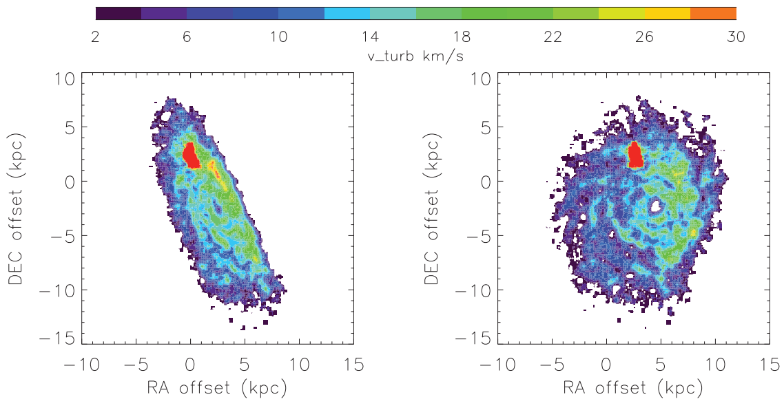
FIGURE 5.42 – Dispersion des vitesses dans le modèle dynamique de NGC 4568.
