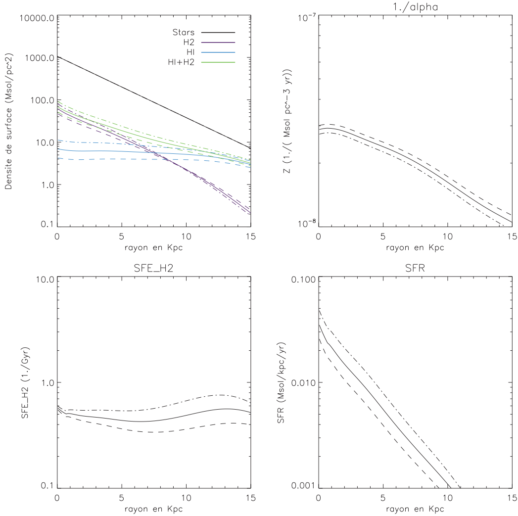
FIGURE 4.4 – Profils radiaux résultants du modèle analytique avec variation de \dot{M} . Haut gauche , les densités de surface de \Sigma_{*} , \Sigma_{HI} , \Sigma_{H_2} , \Sigma_{HI+H_2} . Haut droite , profil radial de la métallicité Z calculée à partir du "closed box model". Bas gauche , efficacité de formation stellaire. Bas droite , taux de formation stellaire. Les résultats réalisés avec le profil Toomre Q présenté dans la figure 4.1, \dot{M} = 0.1 M_{\odot}/yr et \delta = 10 le sont en trait plein. Les lignes en tirets sont réalisées avec le paramètre \dot{M}/2 , les ligne est points tirets sont réalisées avec \dot{M} \times 2 .
