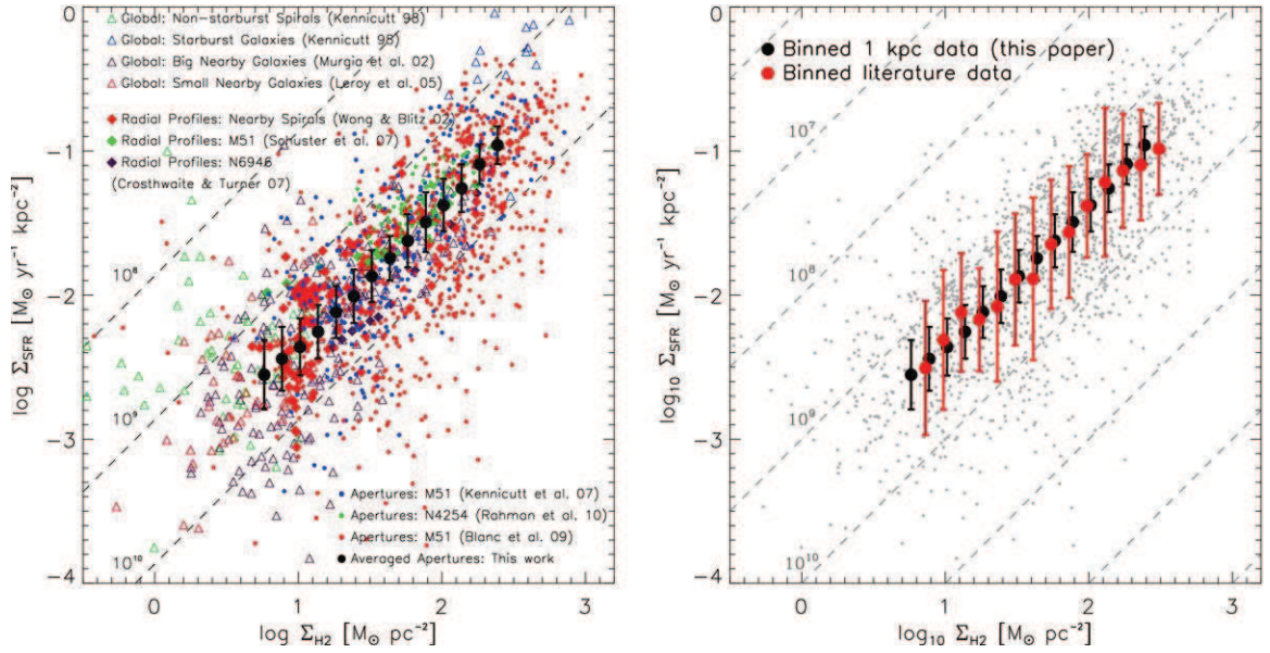
FIGURE 1.3 – Figure (3) de Bigiel et al. (2011). À gauche, le taux de formation stellaire \dot{\Sigma}_* en fonction de la densité de surface du gaz moléculaire \Sigma_{H_2} pour divers relevés, les lignes discontinues obliques montrent différents temps de déplétion du gaz moléculaire. À droite, idem avec les données échantillonnées, les points gris indiquant les mesures individuelles.
