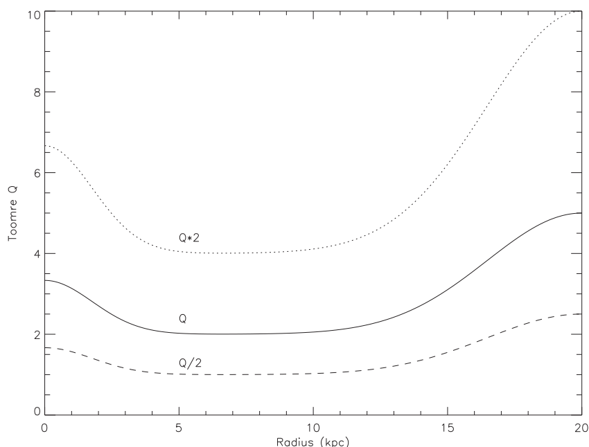
FIGURE 4.1 – Profil radial du paramètre Toomre Q , défini comme paramètre d’entrée du modèle analytique de NGC 4501. En pointillés, le profil de Q \times 2 , en tirets, le profil de Q/2 .
