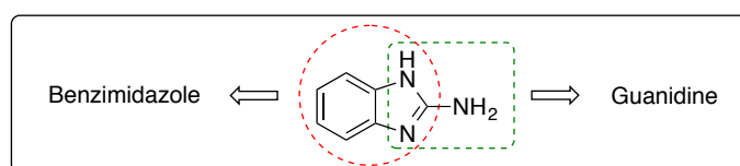
Figure 2-2. Structure du 2-AB
