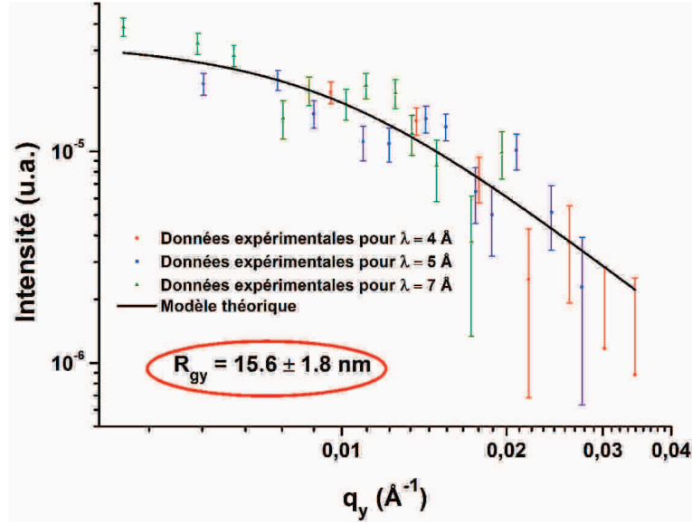
Figure 5: Courbes expérimentales GISANS pour un film multicouche contenant 50% de PSS deutéré. Les données expérimentales (points) pour les longueurs d'onde de 5 Å, 7 Å et 9 Å, ainsi que la fonction de Debye correspondante (ligne) sont représentées.
