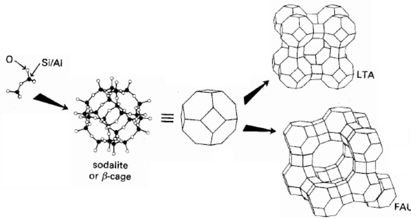
Figure II.1 : Représentation schématique de la structure des zéolithes avec de petits pores (1-20 Å).
