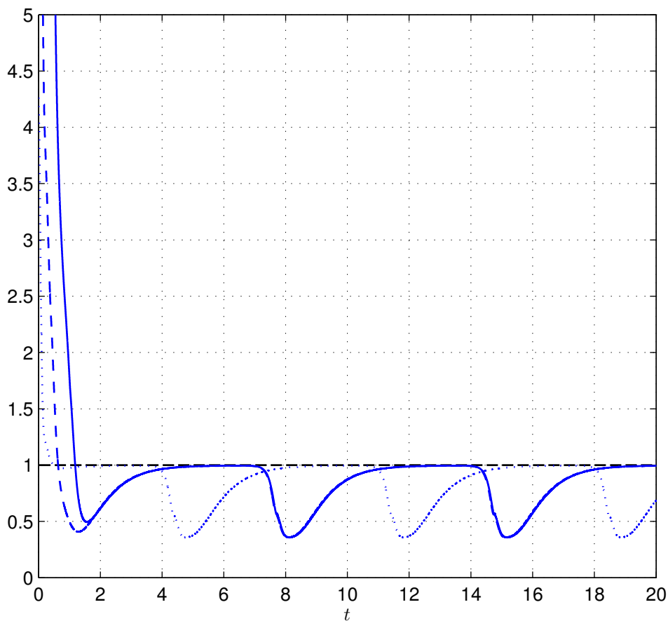
FIGURE 2.2 – L'évolution de la fonction V(x) = x^\top Px . x_0 = (0, \pi/8, 0, 0) (ligne continue), x_0 = (0, \pi/18, 0, 0) (ligne en tirets), x_0 = (0, \pi/36, 0, 0) (ligne pointillée).
