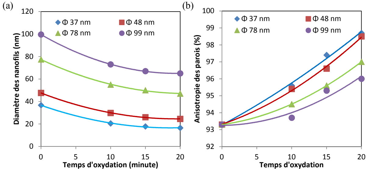
Figure 0.23 – Courbes d'évolution géométrique des réseaux des nanofils en fonction tu temps d'oxydation (a) diamètre des nanofils, (b) anisotropie des parois.
