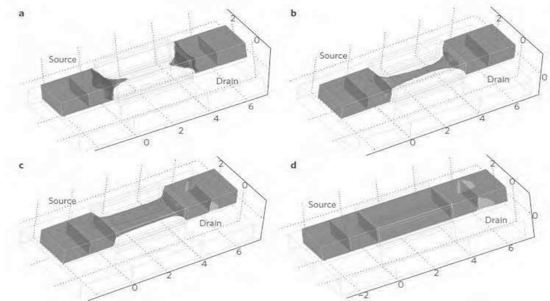
Figure 0.17 – Variation de la concentration d'électrons dans le canal de conduction d'un transistor sans jonction de type n (a) V_g < V_{th} le canal est dépeuplé de porteurs (b) V_g = V_{th} formation du canal de conduction entre la source et le drain (c) V_g > V_{th} expansion du canal de conduction (d) à condition de bande plate, ie V_g = V_{fb} \gg V_{th} le transistor se comporte comme une simple résistance [49].
