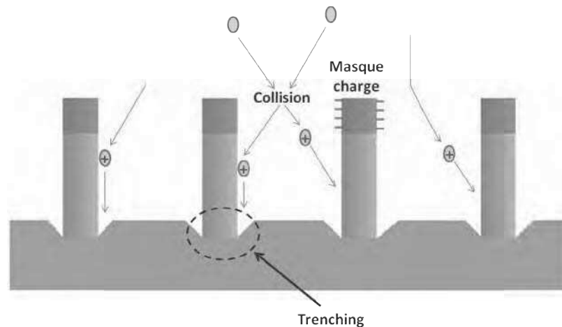
Figure 0.14 – Schéma d'illustration sur le phénomène de tranchée.
