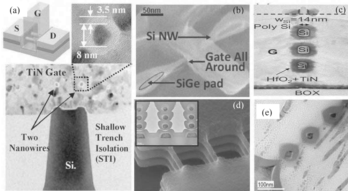
Figure 0.21 – (a- b) Procédé utilisant le SiGe comme couche sacrificielle pour la réalisation des nanofils suspendus par Suk et al. [86] et Coquand et al. [90] respectivement, (c et d) empilement vertical de nanofils en Si suspendus en utilisant le système Si/SiGe par Dupré et al. [94] et Suk et al. [92] respectivement et (e) empilement vertical de nanofils en Si suspendus obtenus par procédé gravure Bosch et oxydation limitée [95].
