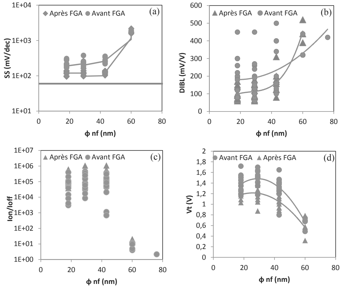
Figure 0.4 – (a) SS (b) DIBL (c) rapport I_{on}/I_{off} et (d) la tension de seuil en fonction du diamètre des nanofils après FGA.
