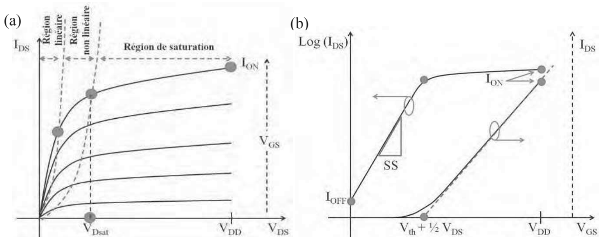
Figure 0.5 –Caractéristiques idéales (a) de sortie ( I_{DS}(V_{DS}) ) et (b) de transfert ( I_{DS}(V_{GS}) ) d'un MOSFET.
