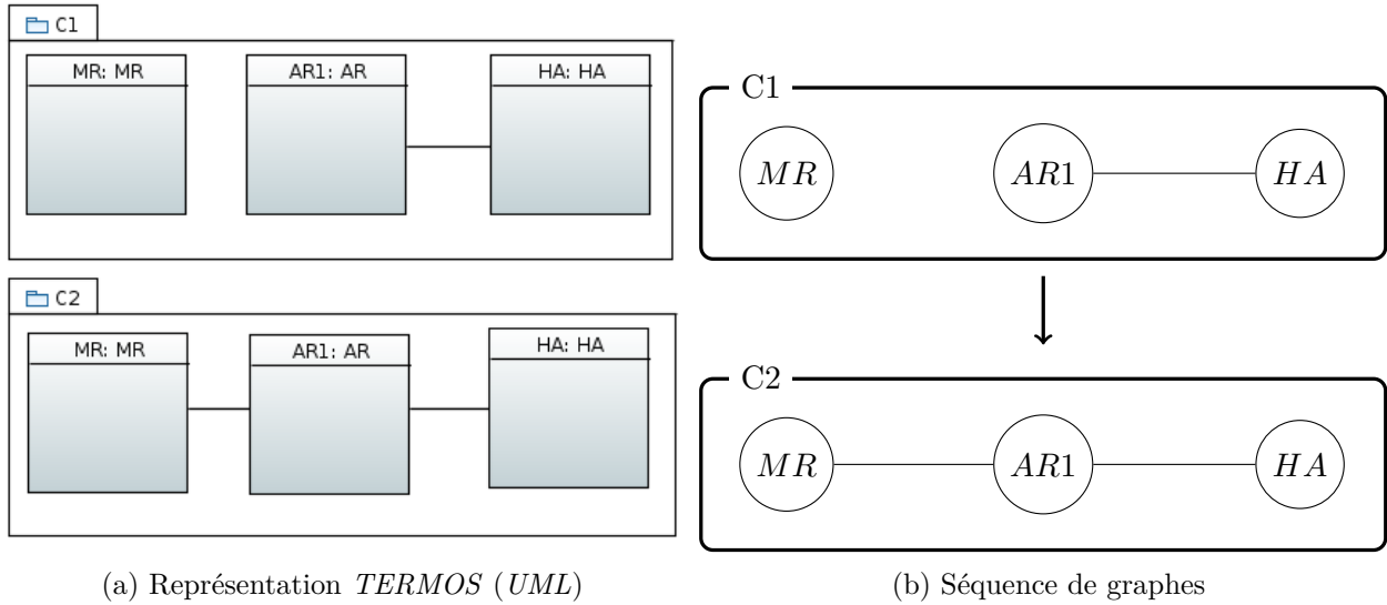
FIGURE 5.10 – Transformation d'une vue spatiale en séquence de graphes
