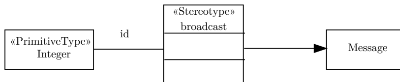
FIGURE 5.6 – Stéréotype appliqué à un message diffusé
