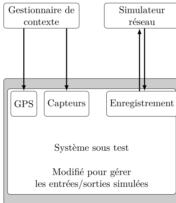
FIGURE 7.2 – Système sous test instrumenté
